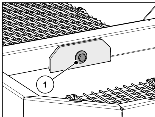
Фиг. 47: Закрепване на разтегателния прът на резервоара
