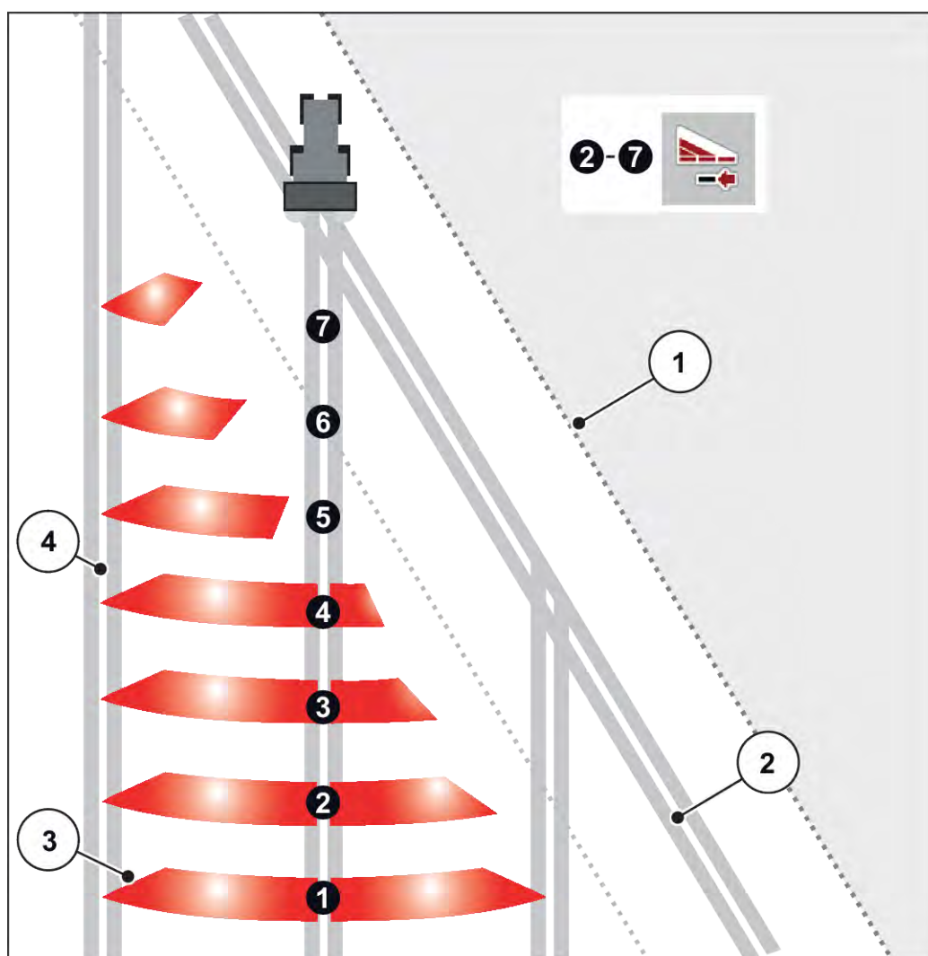
Фиг. 32: Пример за превключване на част от широчината на секцията с VariSpread pro
