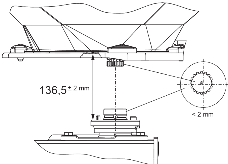
Fig. 52: Kontrollere plassering av spredeskivenav
