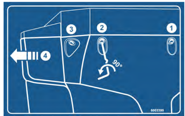
Ábr. 51: Tájékoztató matrica, sárvédő
