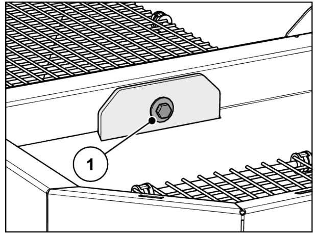
Ábr. 47: A húzórud rögzítése a tartályban
