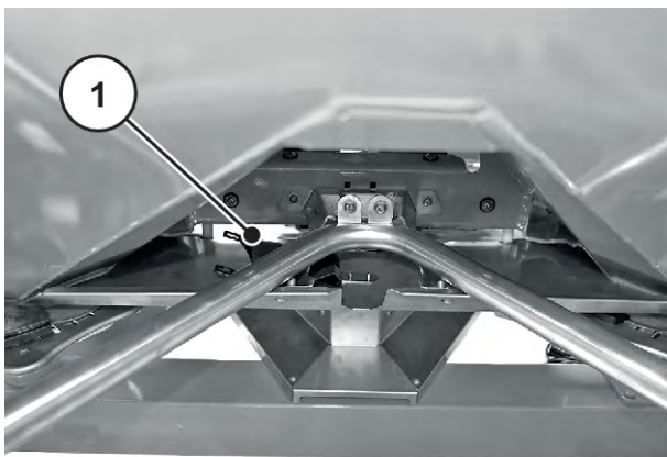
Ábr. 35: A leforgatási próba csúszdája
