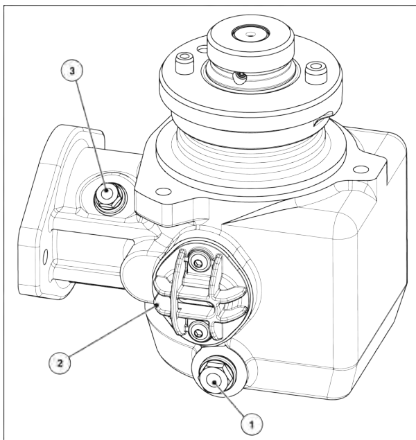
Ábr. 67: Hajtóműolaj betöltési és leeresztési helyei
