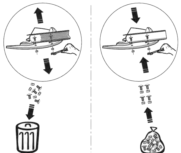
Ábr. 57: Használjon új önzáró anyát
