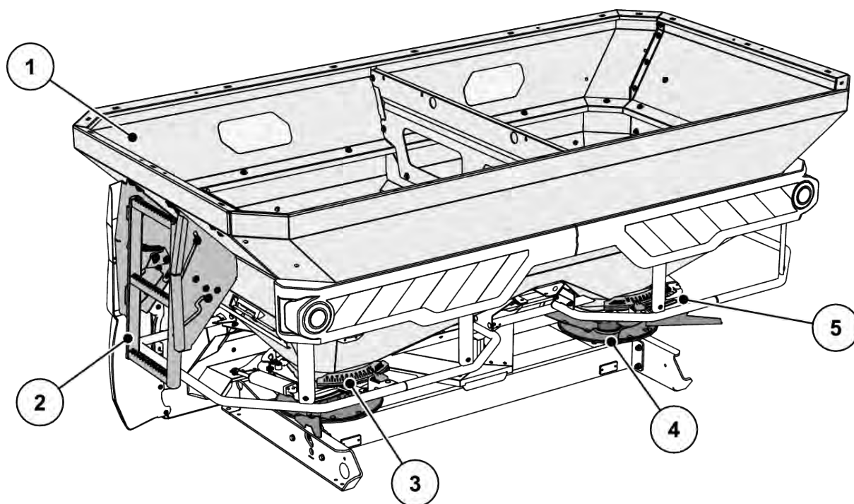
Fig. 6: Komponentgrupsöversikt: Baksida
