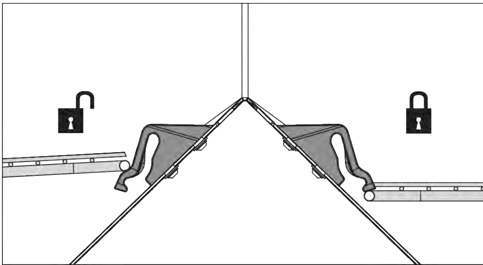
Fig. 48: Skyddsgallerslås öppet/stängt
