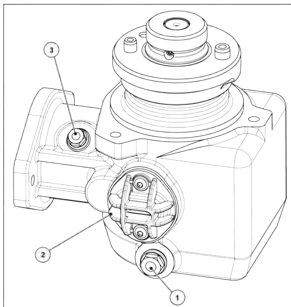
Fig. 67: Påfyllnings- och avtappningsställen för växellådsolja
