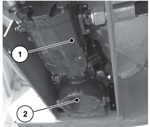
Fig. 65: Hydraulmotor
