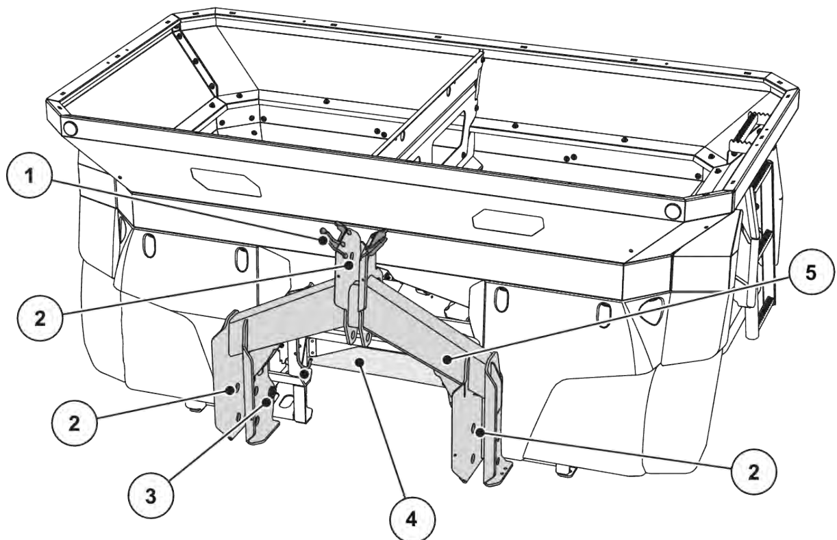
Fig. 5: Komponentgruppöversikt: Framsida
