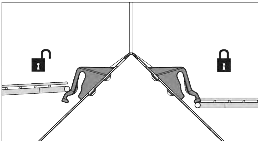
Fig. 48: Skyddsgallerslåsning öppen/stängd
