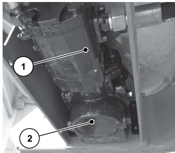
Fig. 65: Hydraulmotor
