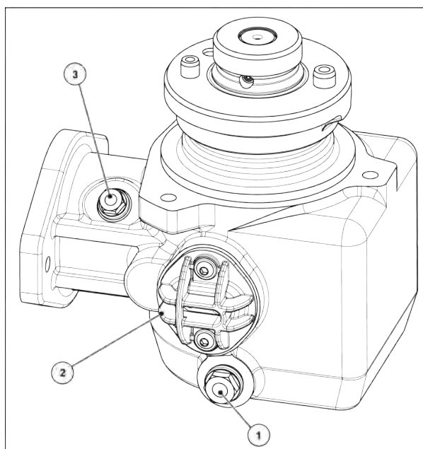
Fig. 67: Påfyllnings- och avtappningsställen för växellådsolja
