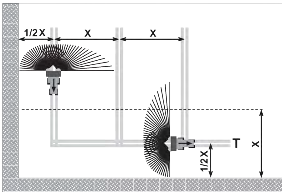
Fig. 30: Gränsspridning
