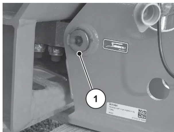
Fig. 64: Smörjpunkt vägningsspridare
