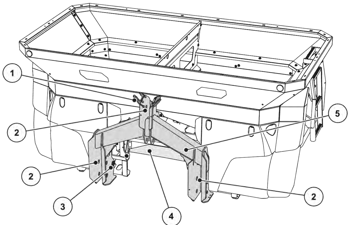
Fig. 5: Komponentgruppöversikt: Framsida
