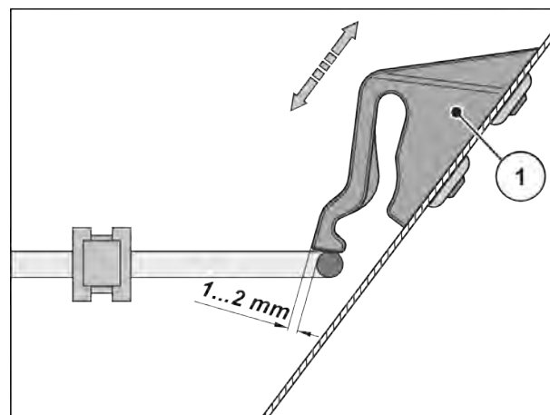
Fig. 50: Cote pentru verificarea funcționării dispozitivului de blocare a grilajului de protecție
