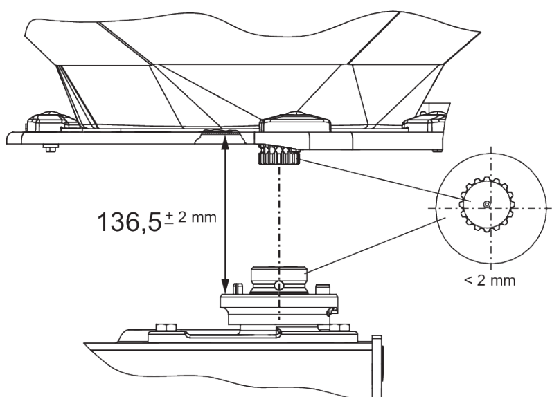
Fig. 52: Verificarea poziției butucului discului aruncător
