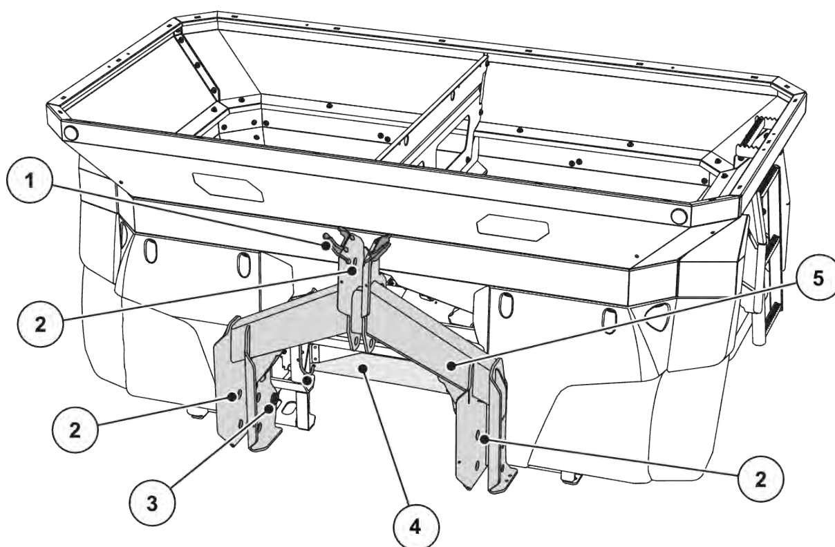
Afb. 5: Module-overzicht: Voorzijde
