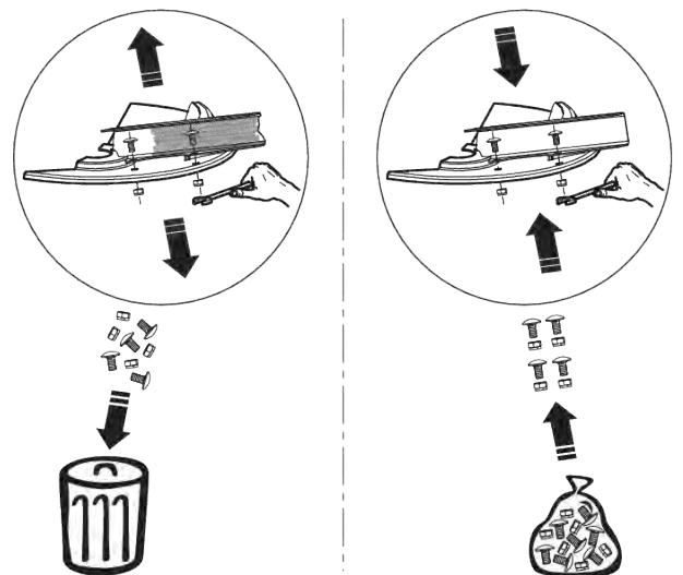
Afb. 57: Nieuwe zelfborgende moeren gebruiken
