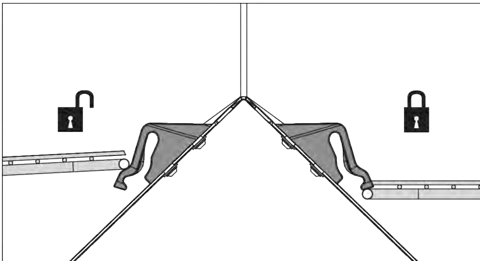
Afb. 48: Beschermroostervergrendeling open/gesloten
