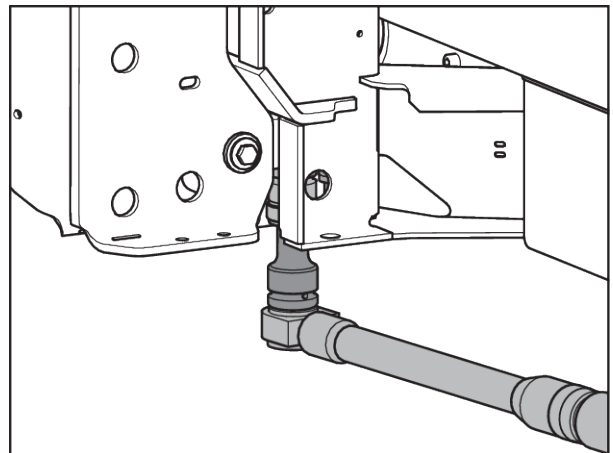
Afb. 45: Bevestiging van de weegcel (in rijrichting links)
