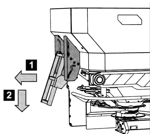
Fig. 43: Klap stigen ud
