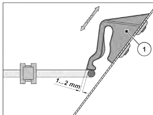
Fig. 50: Kontrolmål til funktionskontrol af beskyttelsesgitterlåsen
