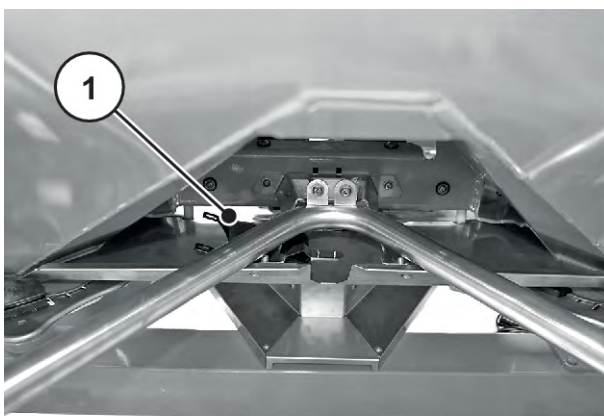
Fig. 35: Kalibreringsprøvesliske
