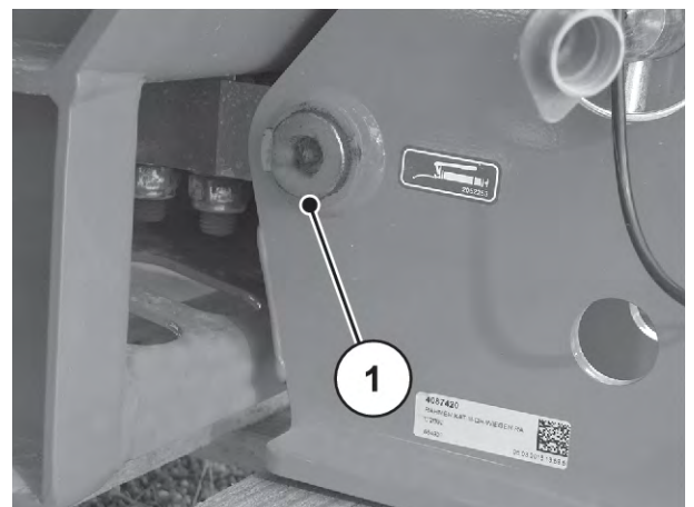
Fig. 64: Point de lubrification sur l'épandeur à pesée
