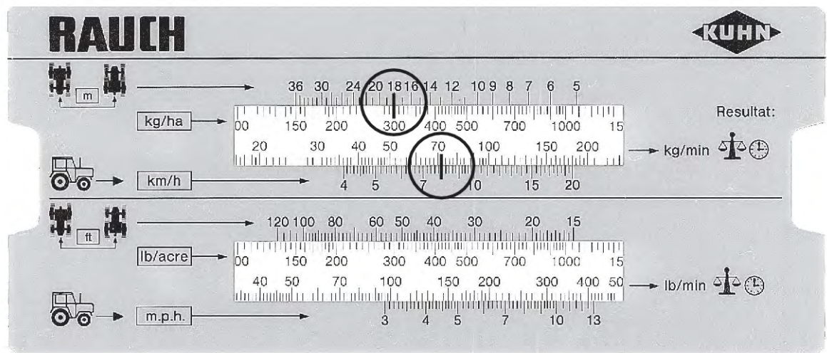
Fig. 34: Echelle pour le calcul théorique de la quantité écoulee par minute
