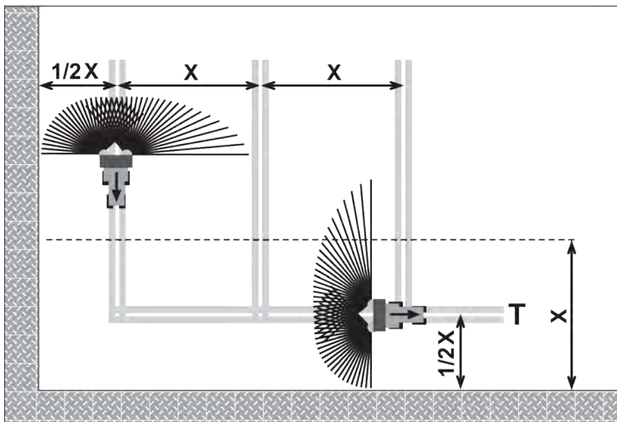
Abb. 30: Grenzstreuen
