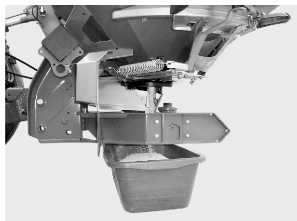
Abb. 38: Abdrehprobe durchführen
