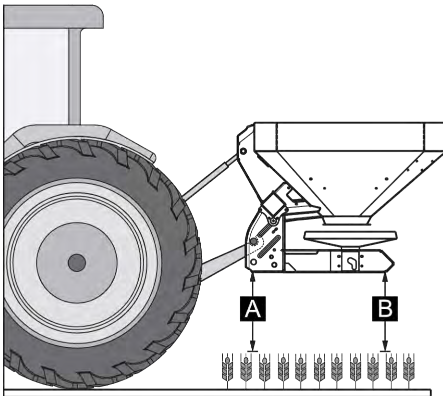
Abb. 12: Anbauposition
