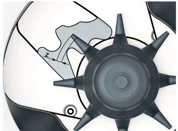
Abb. 54: Verschleißbereich des Rührkopfs
