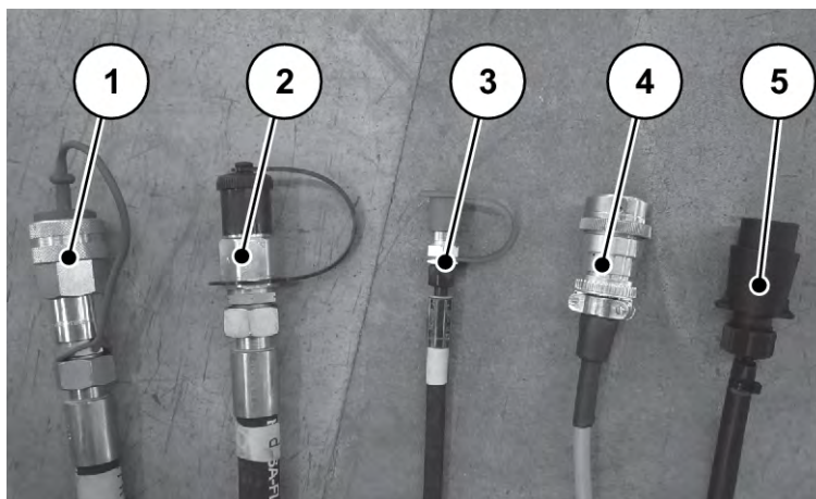
Abb. 13: Anschlussleitungen Wurf-Mineraldüngerstreuer
