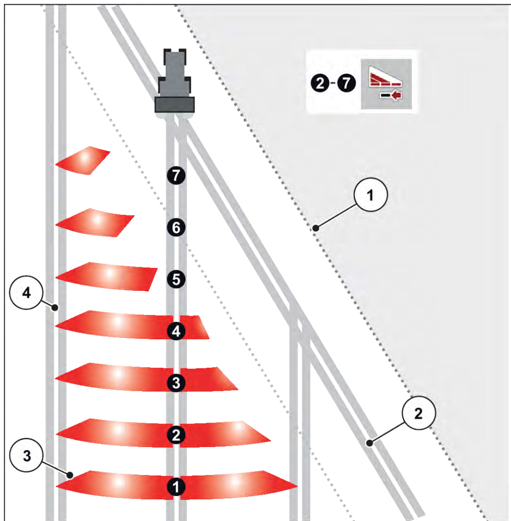
Abb. 32: Beispiel Teilbreitenschaltung mit VariSpread pro
