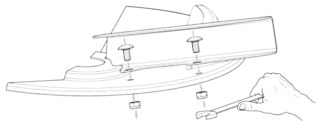
Abb. 56: Schrauben der Wurfweite lösen
