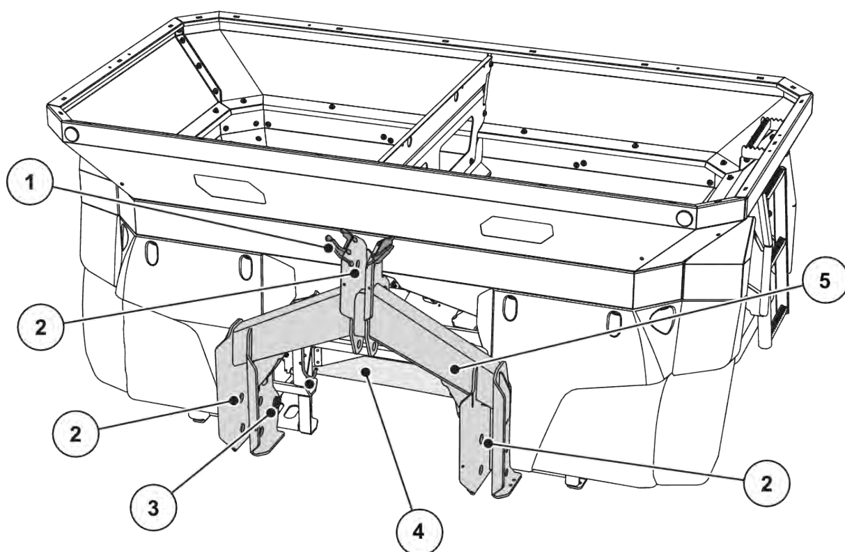
Abb. 5: Baugruppenübersicht: Vorderseite
