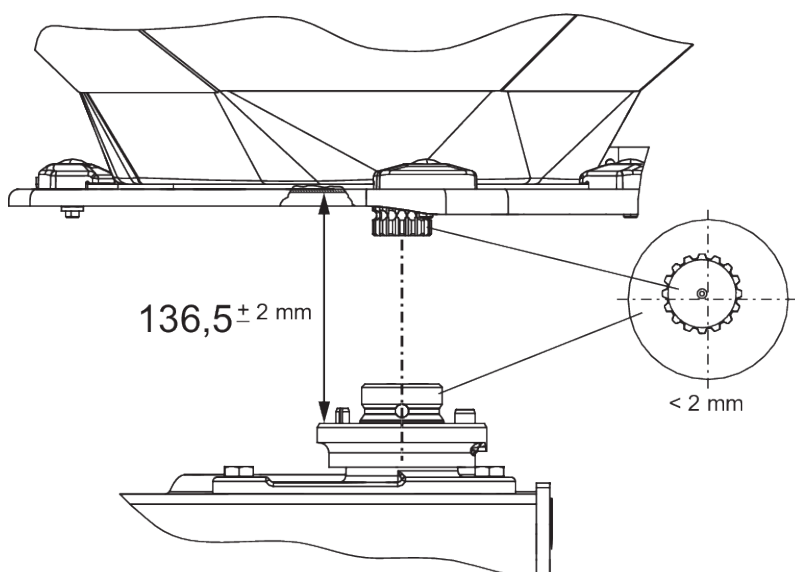
Ilust. 52: Verificar a posição do cubo do disco dispersor
