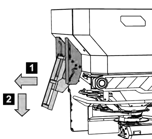
Ilust. 43: Abrir o degrau de subida
