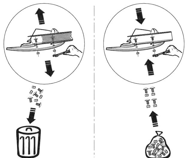
Ilust. 57: Utilizar novas porcas autorroscentes
