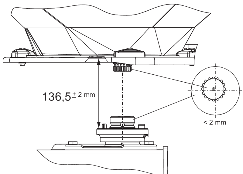
Sl. 53: Provjera glavčine diska za rasipanje
