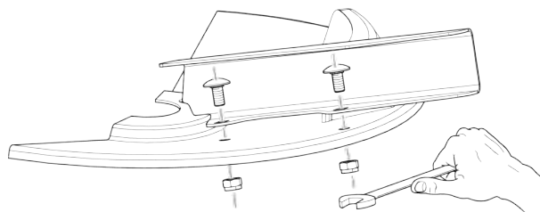
Sl. 57: Otpuštanje vijaka lopatice
