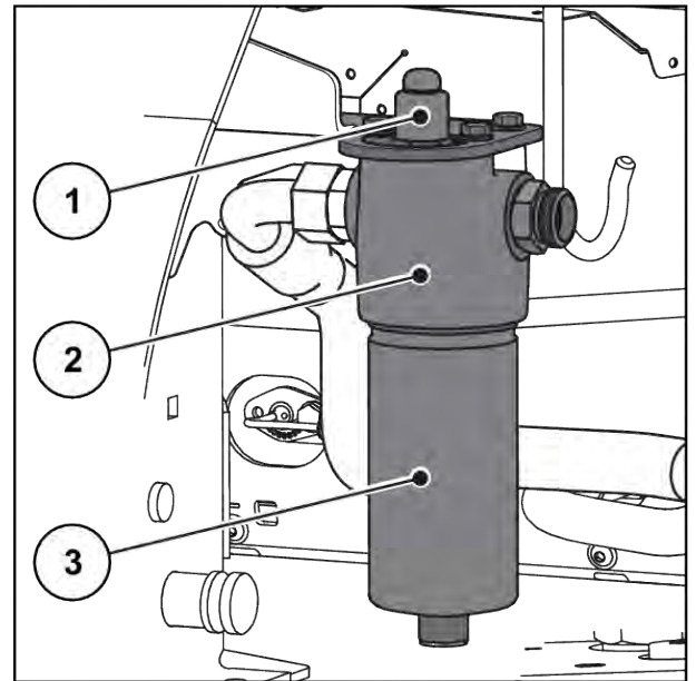
Σχ. 67: Φίλτρο πίεσης υδραυλικού συστήματος
