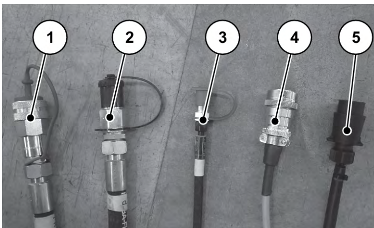
Sl. 12: Priključne napeljave iz metalnega trosilnika mineralnega gnojila
