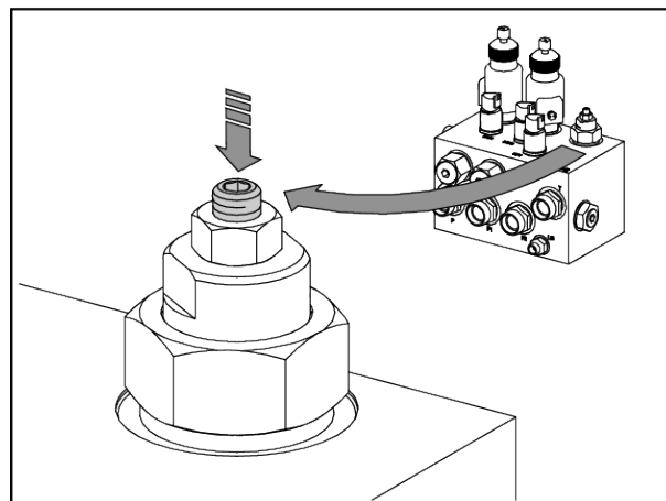
Sl. 14: Nastavitveni vijak na hidravličnem sklopu nastavite na LS
