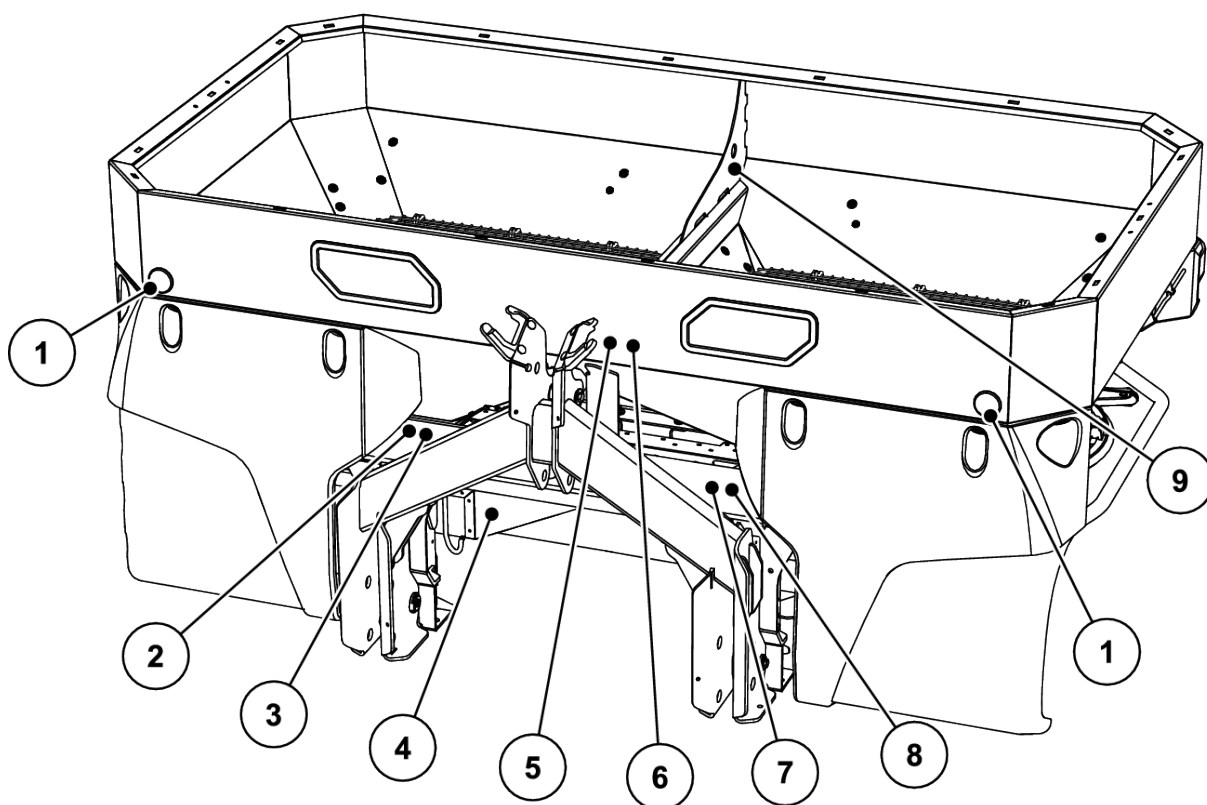
Jn. 2: Kaitseeadised, hoiatus- ja instruksioonijuhiste kleebised, esikülg
