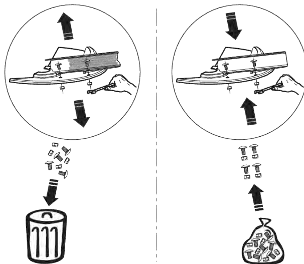
Jn. 58: Uute iselukustuvate mutrite kasutamine
