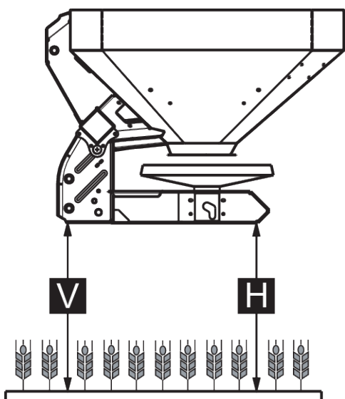
Att. 15: Maksimālais pieļaujamo uzkabšanās augstums normālai un vēlai mēslošanai
