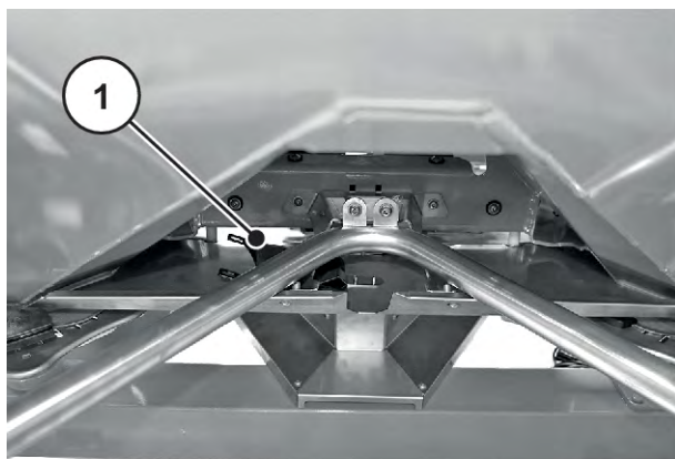
Att. 36: Dozēšanas izmēģinājuma rene
