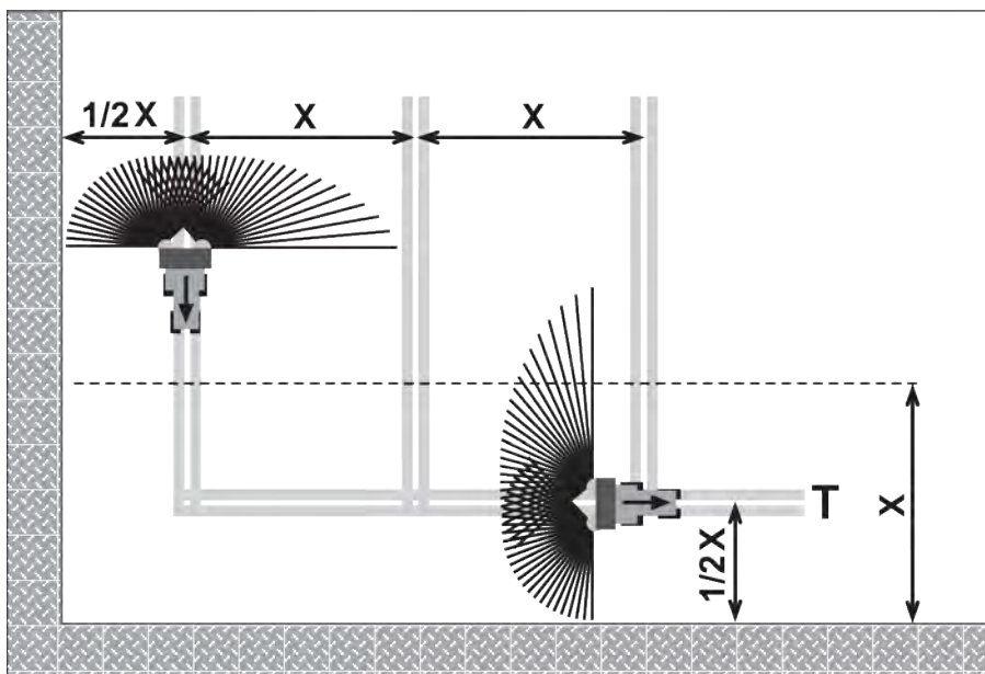
Pav. 31: Paribių barstymas
