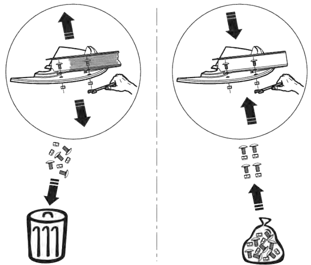
Pav. 58: Naudokite naujas savaime užsifiksuojančias veržles.
