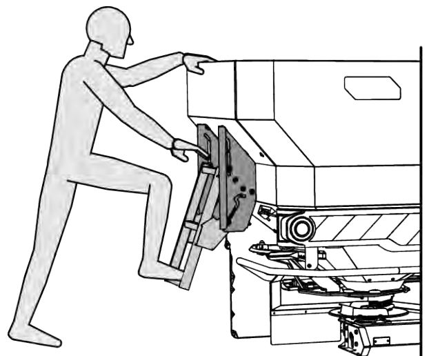
Pav. 42: Kopėčios be rezervuaro dengiamojo tento
