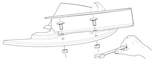
Pav. 57: Atlaisvinkite barstomųjų menčių varžtus.
