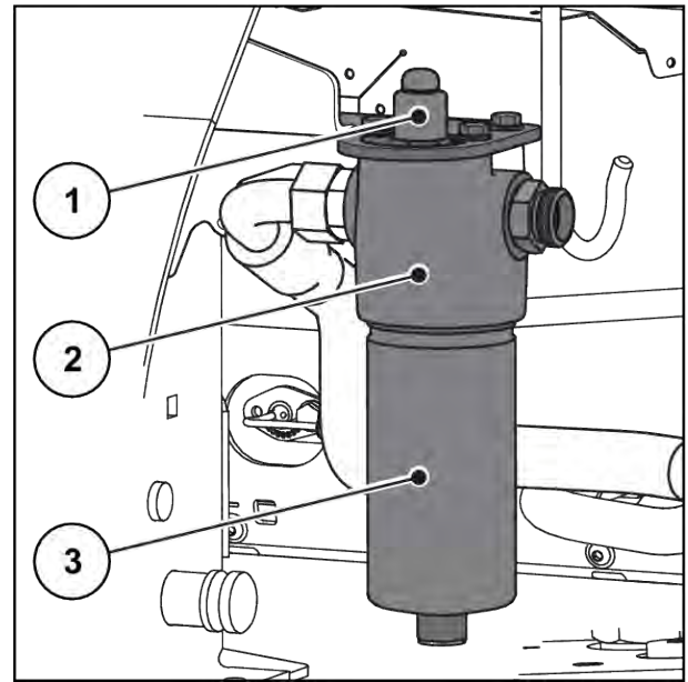
Obr. 67: Hydraulický tlakový filter
