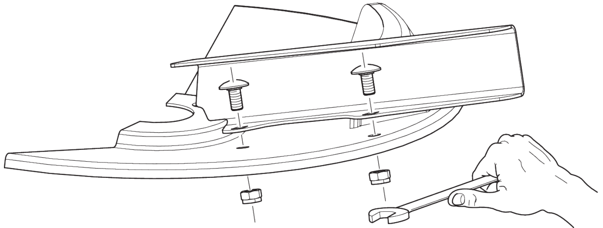
Obr. 57: Povoľenie skrutiek rozmetávacích lopatiek
