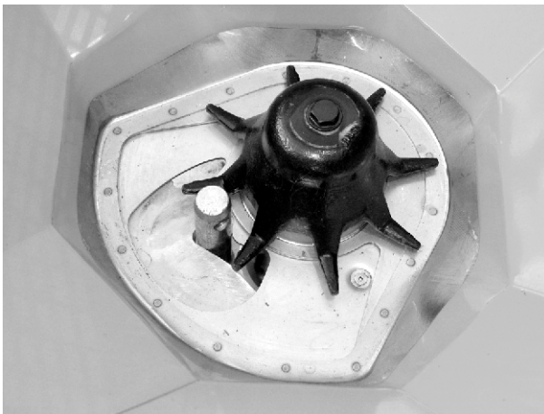
Obr. 59: Čap dolného ramena v dávkovacom otvore
