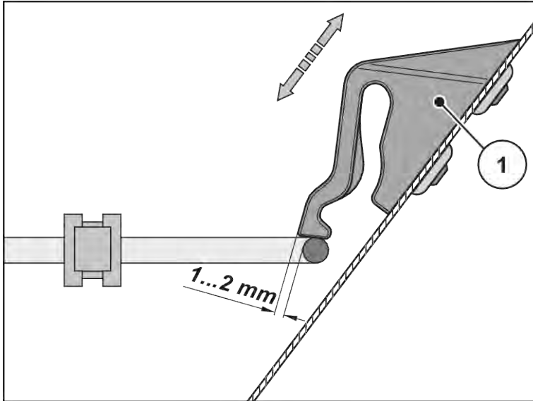
Obr. 51: Mierka na kontrolu funkčnosti zablokovania ochrannej mreže
