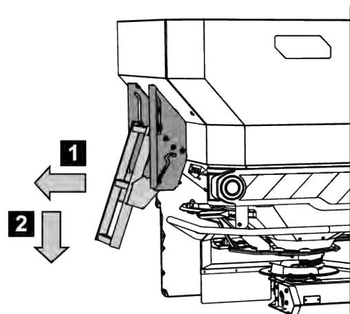
Фиг. 44: Разгъване на стълбата
