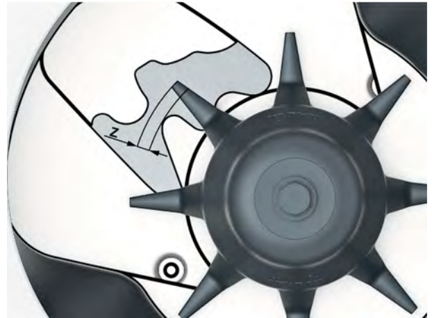
Фиг. 55: Износена зона на главата на смесителния механизъм
