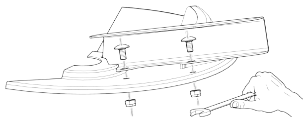
Фиг. 57: Разхлабете винтовете на разпръскващите лопатки
