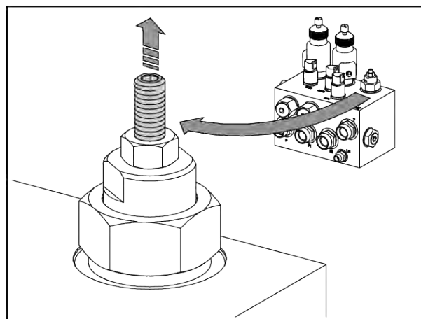
Фиг. 13: Регулиращ винт на хидравличния болт развит за режим KS
