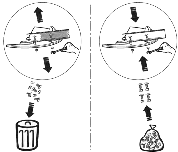
Фиг. 58: Използвайте нови самозаконтрящи се гайки
