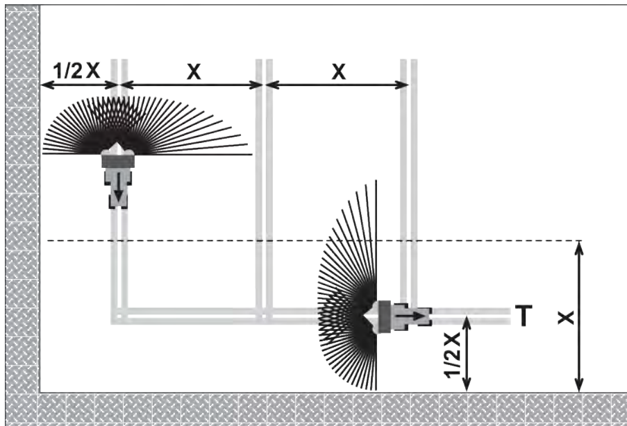
Fig. 31: Grensespredning
