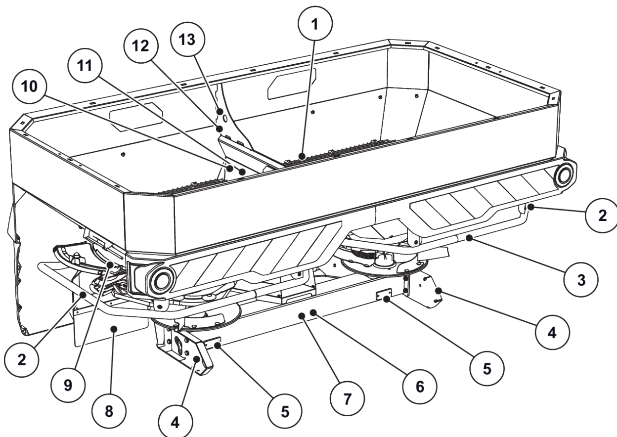
Fig. 3: Beskyttelsesinnretninger, klistremarker advarsler og instruksjonsanvisninger, bakside
