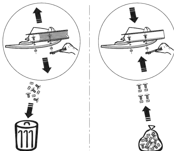
Fig. 58: Bruk nye selvlåsende muttere
