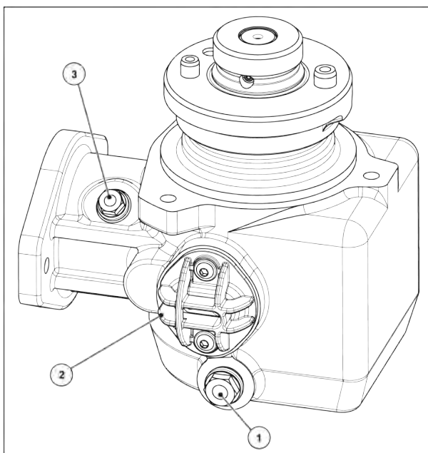
Fig. 68: Fylle- og tappesteder for girolje
