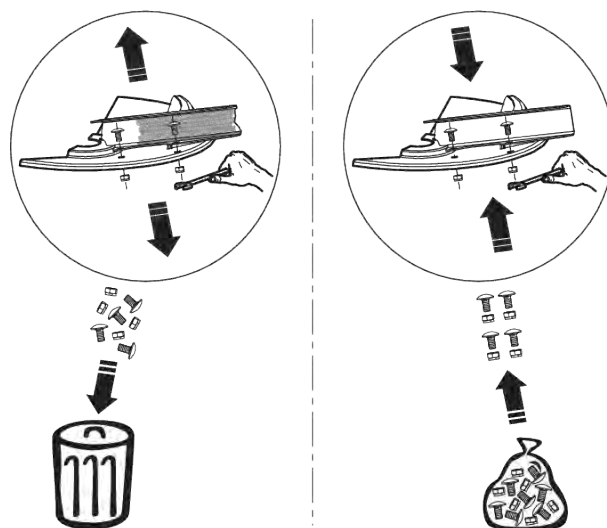
Ilust. 58: Utilizar tuercas nuevas de autobloqueo
