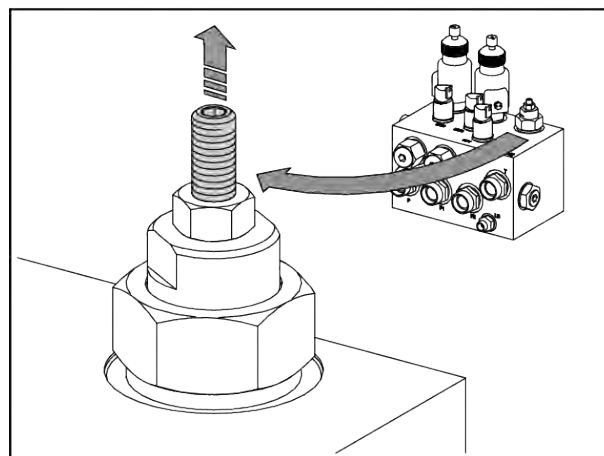
Ilust. 13: El tornillo de ajuste se ha desatornillado del bloque hidráulico para la corriente continua.
