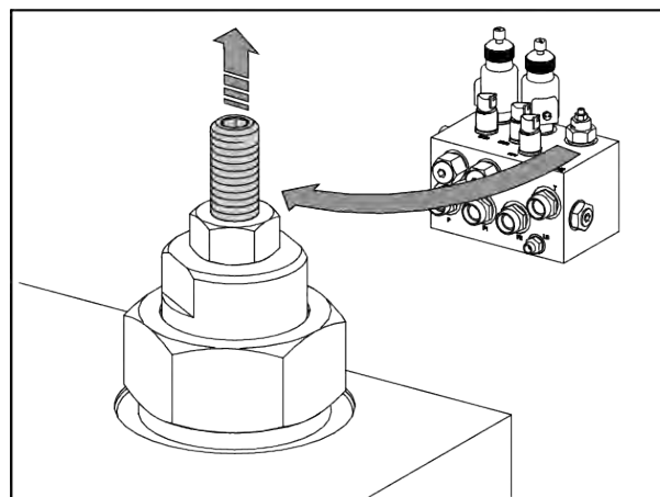
Ábr. 13: A hidraulikablokk állítócsavarja az állandó térfogatáramhoz ki van csavarva
