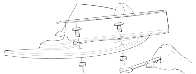
Kuva 57: Levityssiiven ruuvien irrotus
