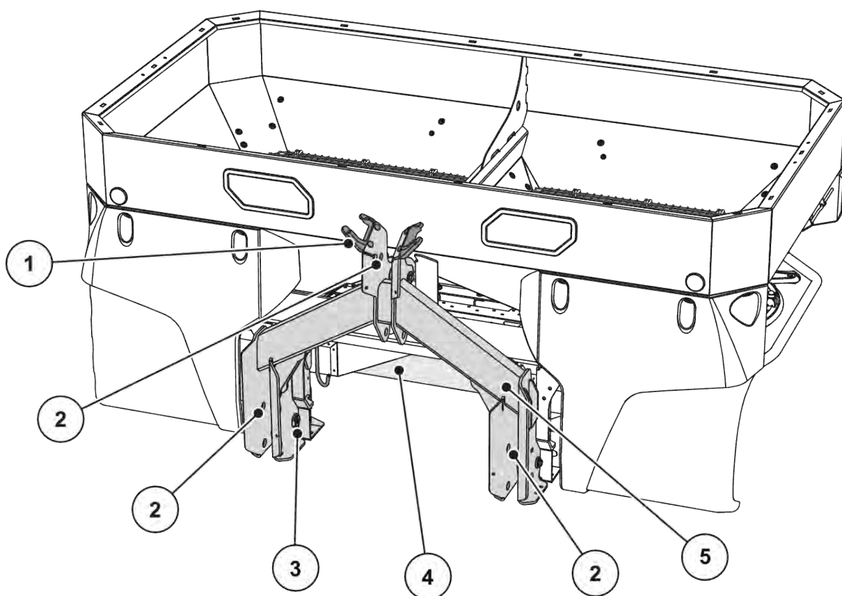
Kuva 5: Rakenneryhmäkuva: Etupuoli
