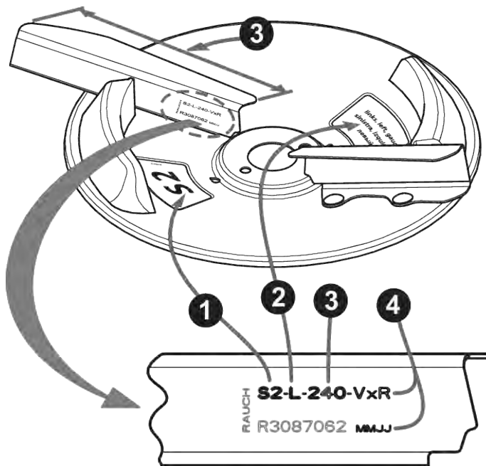
Kuva 56: Levityslautasen teksti
