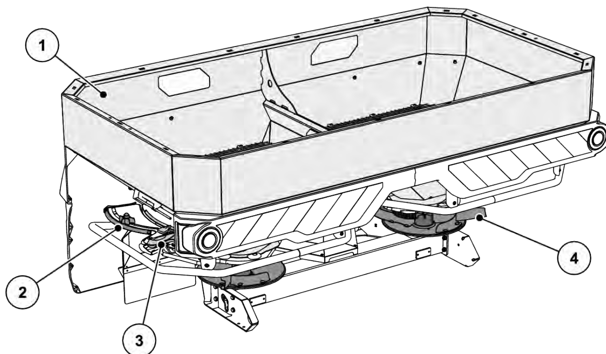
Kuva 6: Rakenneryhmäkuva: Takasivu
