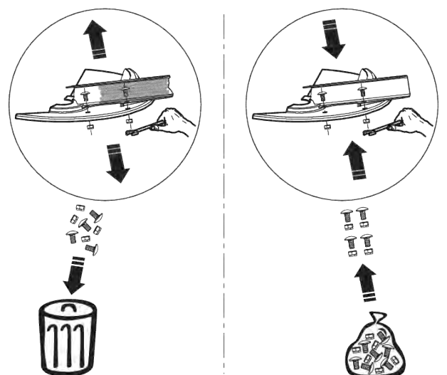
Kuva 58: Uusien itselukittuvien mutterien käyttö
