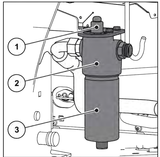
Kuva 67: Hydraulinen painesuodatin
