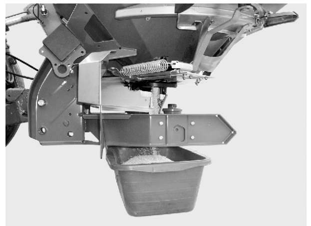
Kuva 39: Kiertokokeen suoritus
