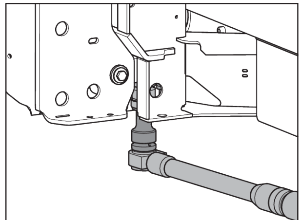
Kuva 46: Punnituskentön kiinnitys (ajosuuntaan nähden vasemmalle)
