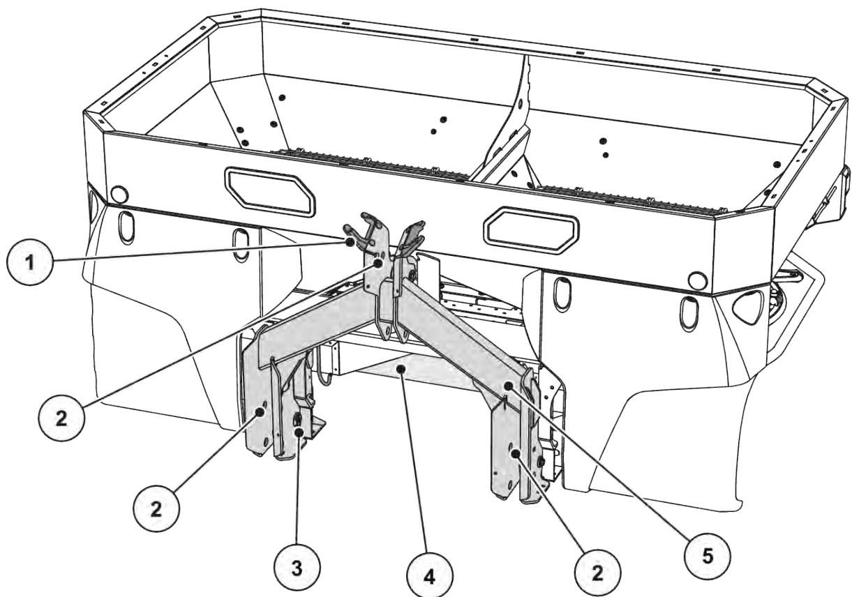
Fig. 5: Komponentgruppöversikt: Framsida
