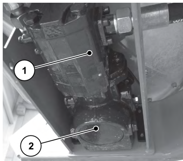
Рис. 66: Гидравлический двигатель
