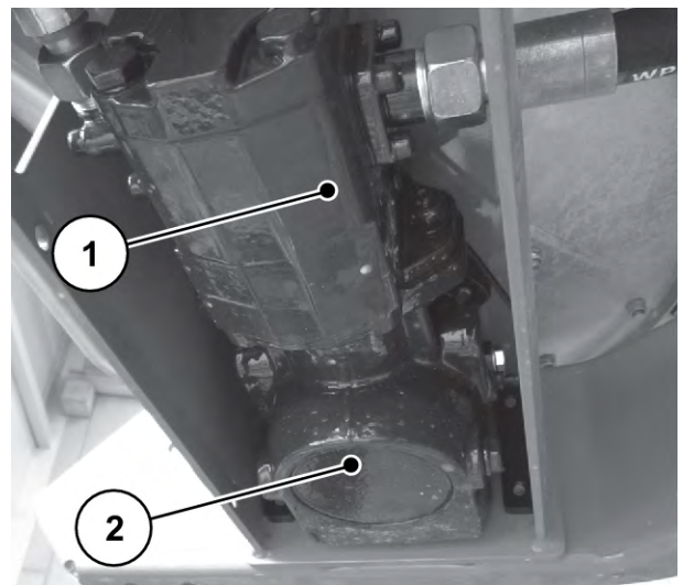
Рис. 66: Гидравлический двигатель
