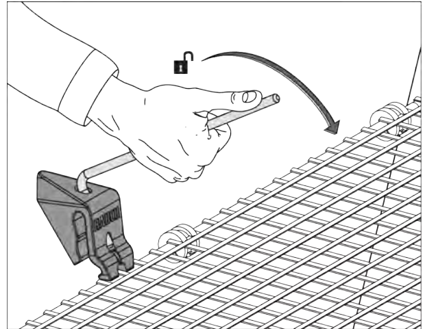
Rys. 50: Otwieranie blokady kratki ochronnej
