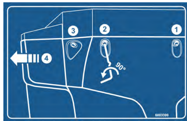
Rys. 52: Naklejka informacyjna: osłony przeciwbłotne
