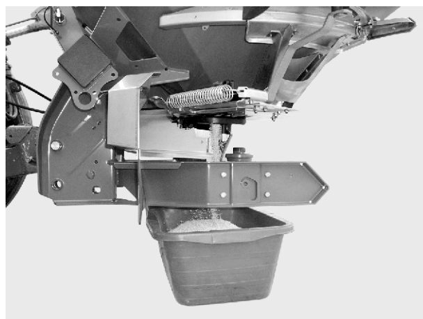
Afb. 39: Afdraairoef uitvoeren
