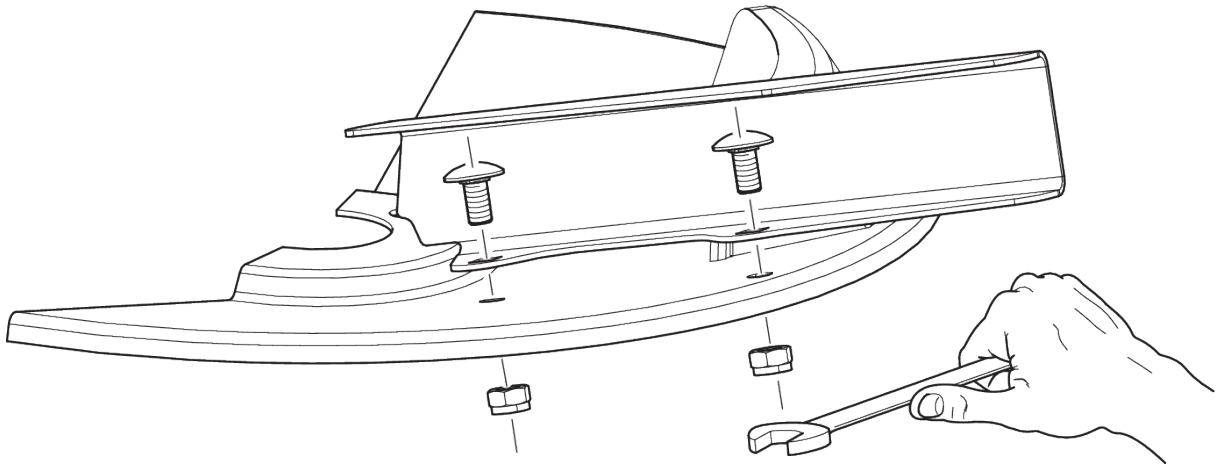
Afb. 57: Schroeven van de stroischoepen losdraaien
