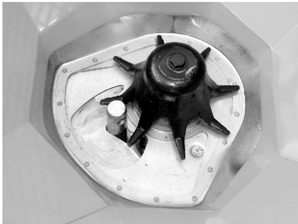
Afb. 59: Bout voor de onderste hefarm in doseeropening
