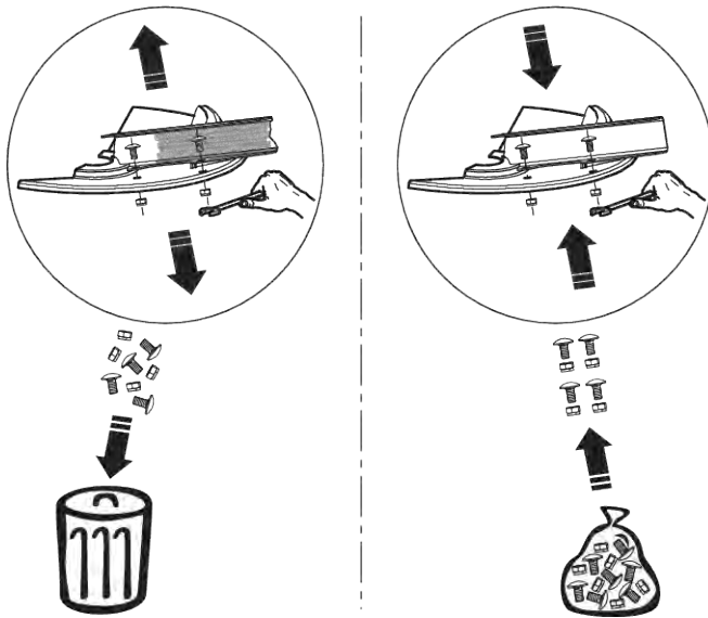
Afb. 58: Nieuwe zelfborgende moeren gebruiken
