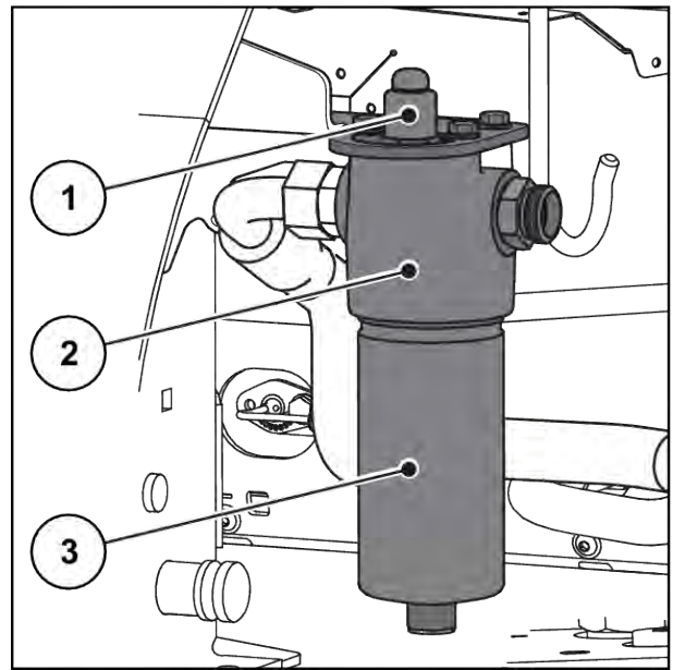
Afb. 67: Hydraulisch drukfilter
