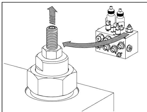
Afb. 13: Stelschroef aan het hydraulische blok voor CS uitgedraaid.
