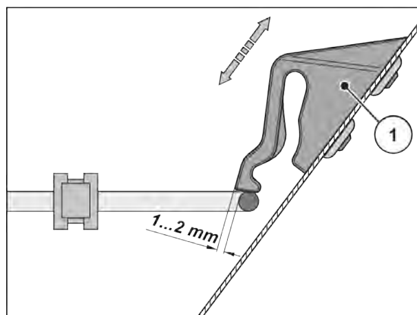
Fig. 51: Kontrolmål til funktionskontrol af beskyttelsesgitterlåsen
