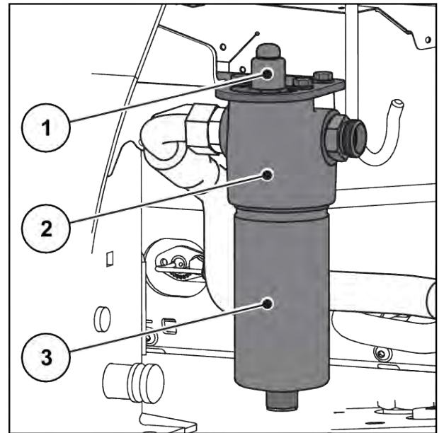
Fig. 67: Hydrauliktrykfilter
