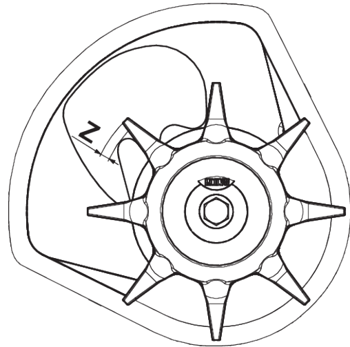
III. 55: Limite di usura della testa dell'agitatore
