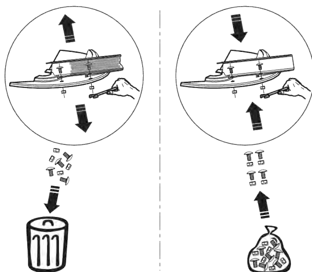
III. 58: Utilizzo di dadi autobloccanti nuovi
