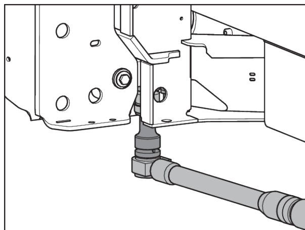
III. 46: Fissaggio della cella di pesatura (a sinistra, nel senso di marcia)
