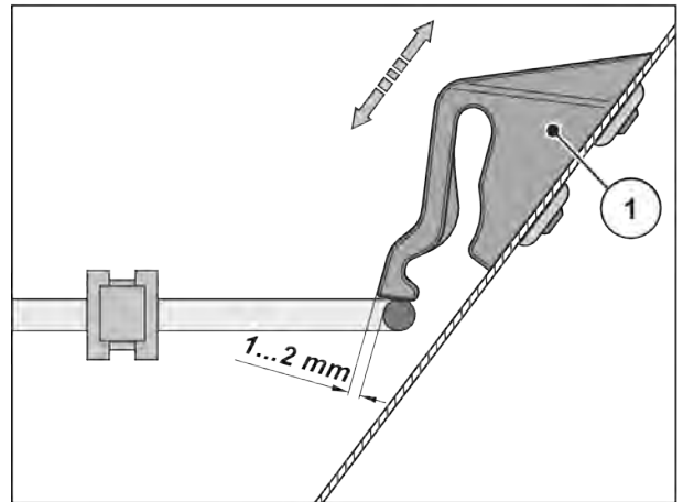
III. 51: Misura per il controllo del funzionamento del bloccaggio della griglia protettiva
