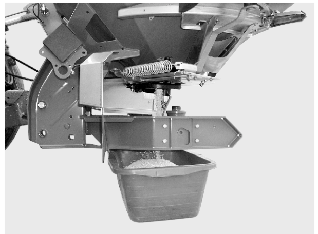
Fig. 39: Effectuer un test d'épandage
