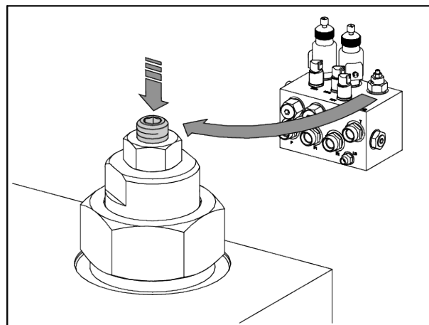
Fig. 14: Ajuster la vis de réglage du bloc hydraulique pour LS
