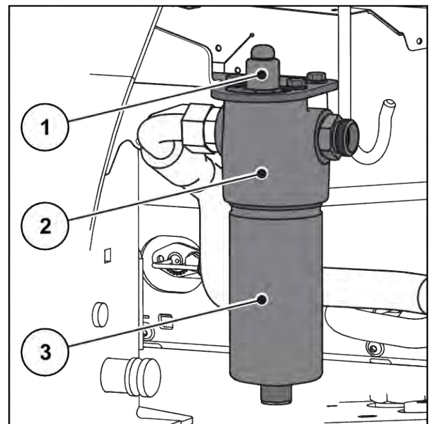
Abb. 67: Hydraulik Druckfilter
