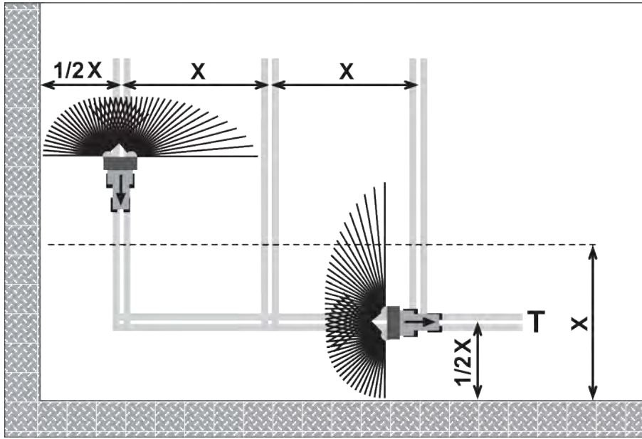
Şek. 31: Sınır serpme
