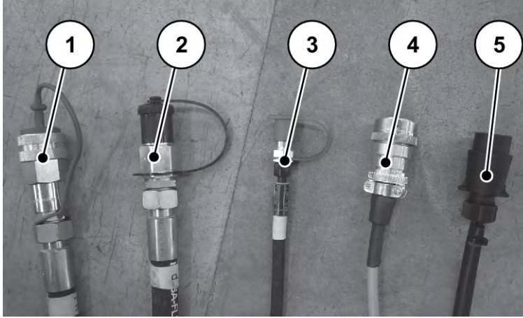
Şek. 12: Mineral gübre serpme makinesi bağlantı hatları
