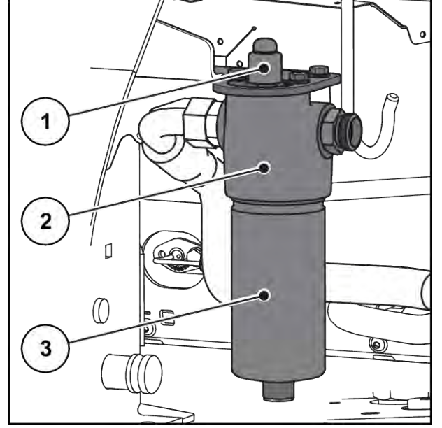
Şek. 67: Hidrolik basınç filtresi
