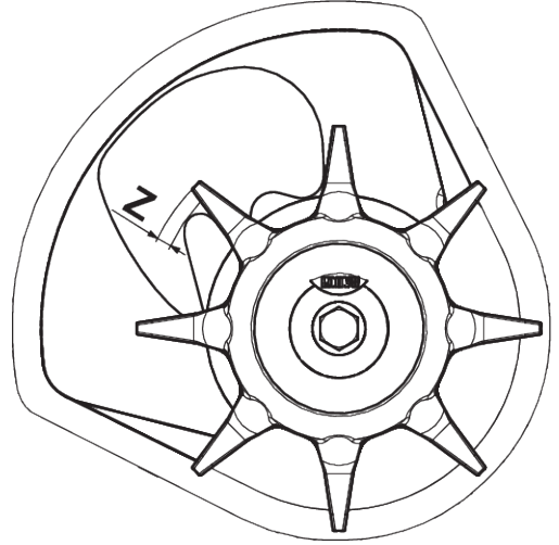
Şek. 55: Karıştırıcı kafasının aşınma bölgesi
