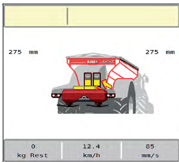
Rys. 8: Czujnik stanu napełnienia zbiornika AXENT
