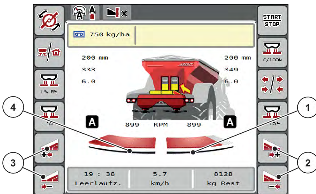
Rys. 38: Ekran roboczy: Szerokości częściowe z 2 stopniami
