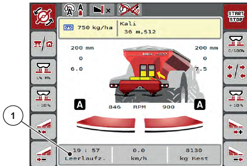
Rys. 42: Wskazanie pomiaru biegu jałowego na ekranie roboczym
