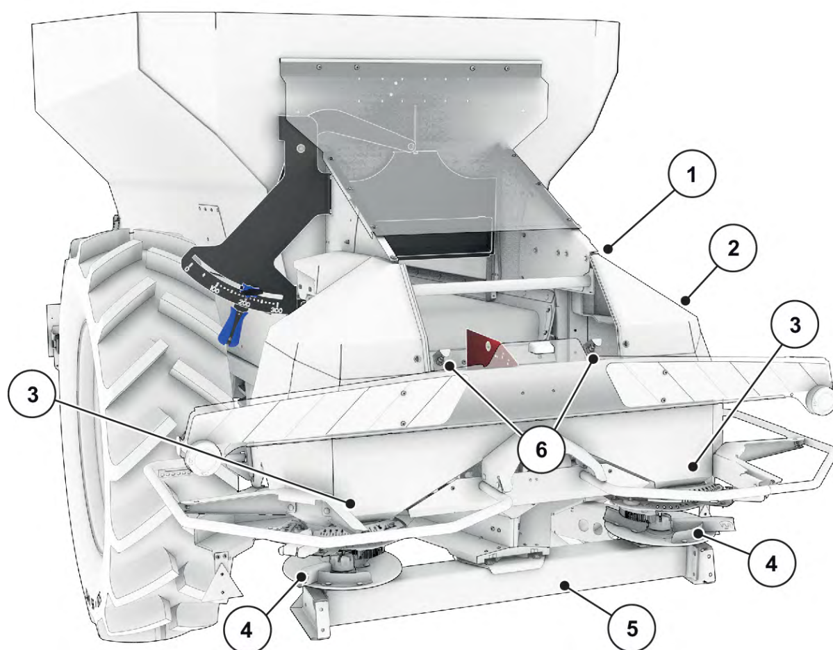
Rys. 6: Przegląd urządzeń wykonawczych i czujników w rozsiewaczu wielkopowierzchniowym AXENT i rozrzutniku nawozu
