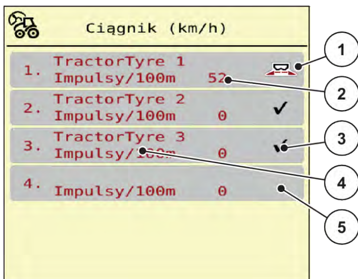
Rys. 21: Menu Ciągnik (km/h)
