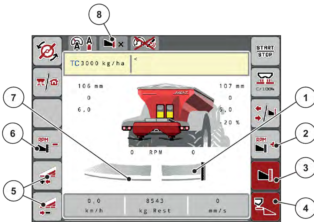
Rys. 40: Ekran roboczy z jedną szerokością częściową po lewej stronie i wysiewem granicznym po prawej stronie
