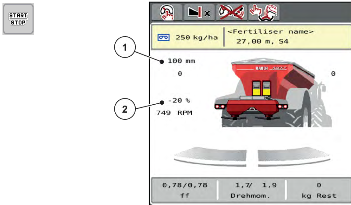
Rys. 43: Ekran roboczy MAN Skala
