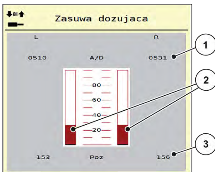
Rys. 26: Test/diagnostyka; przykład: Zasuwa dozująca
