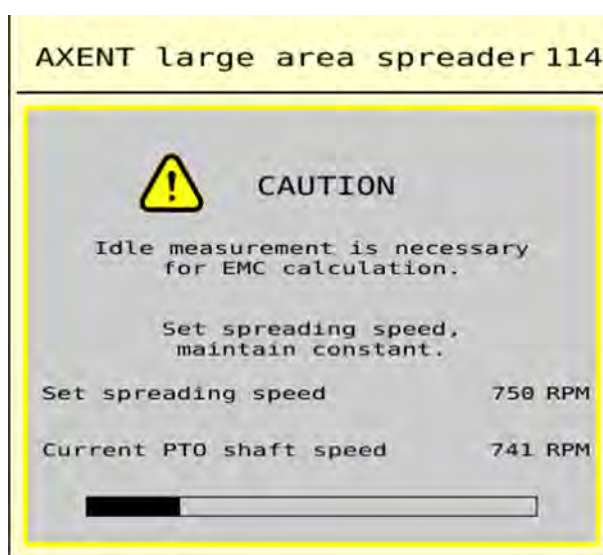
Rys. 41: Wyświetlanie alarmów pomiaru biegu jałowego
