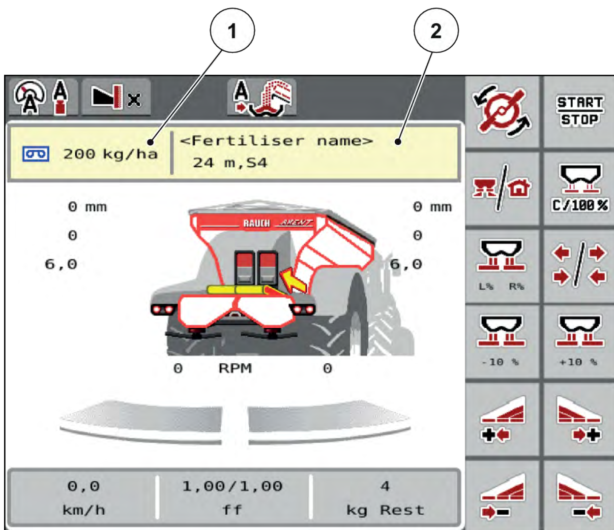
Rys. 12: Wprowadzanie dawki wysiewu na ekranie dotykowym
