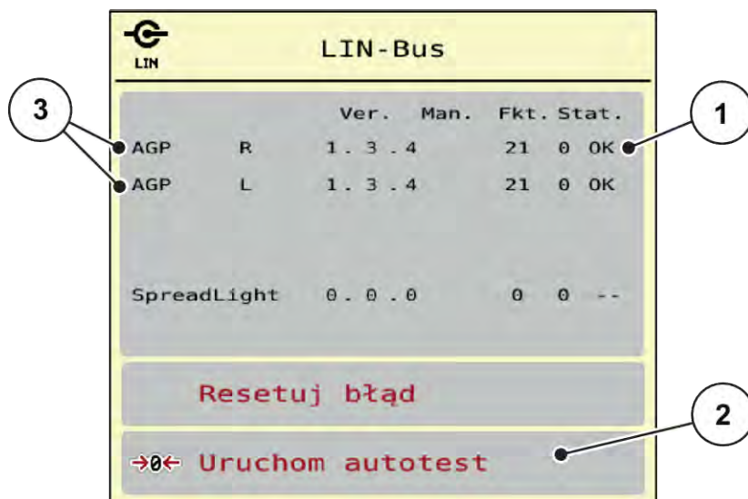
Rys. 27: System/test; przykład: Test/diagnostyka
