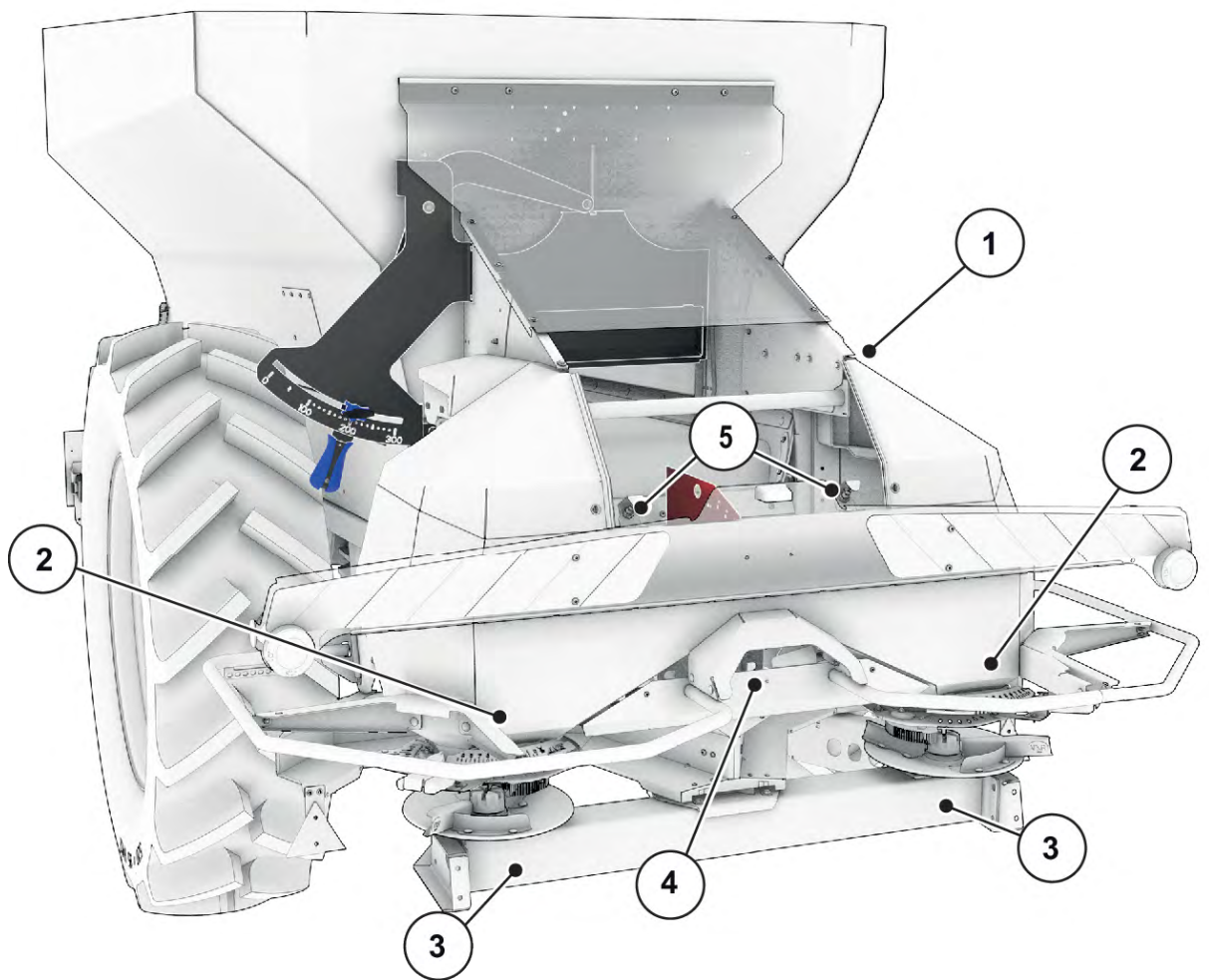
Abb. 6: Übersicht der Aktoren und Sensoren am Großflächenstreuer AXENT und Düngerstreuwerk
