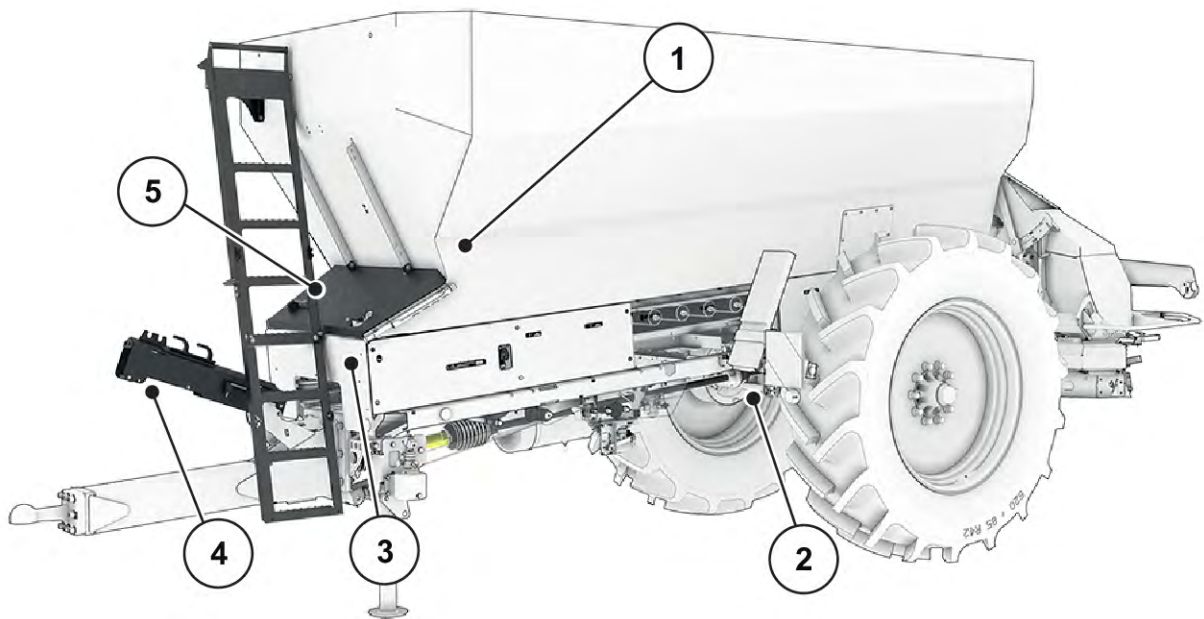
Abb. 5: Übersicht der Aktoren und Sensoren am Großflächenstreuer AXENT
