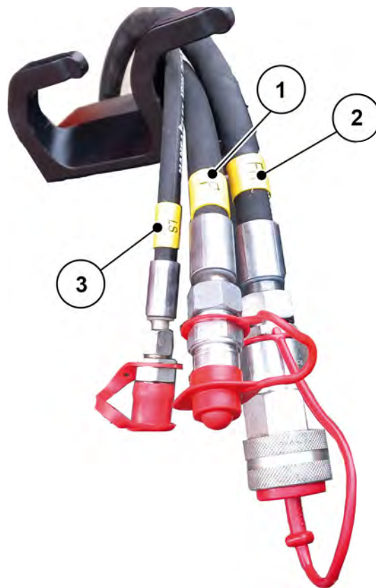
Obr. 24: Označení hydraulických hadic
