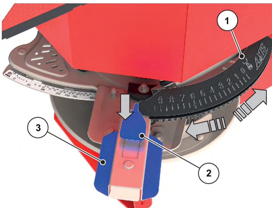
Obr. 44: Centrum pro nastavení bodu výpadu
