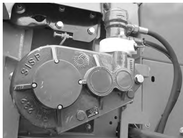
Obr. 71: Kontrola motoru a hydraulického bloku pohonu dopravního pásu
