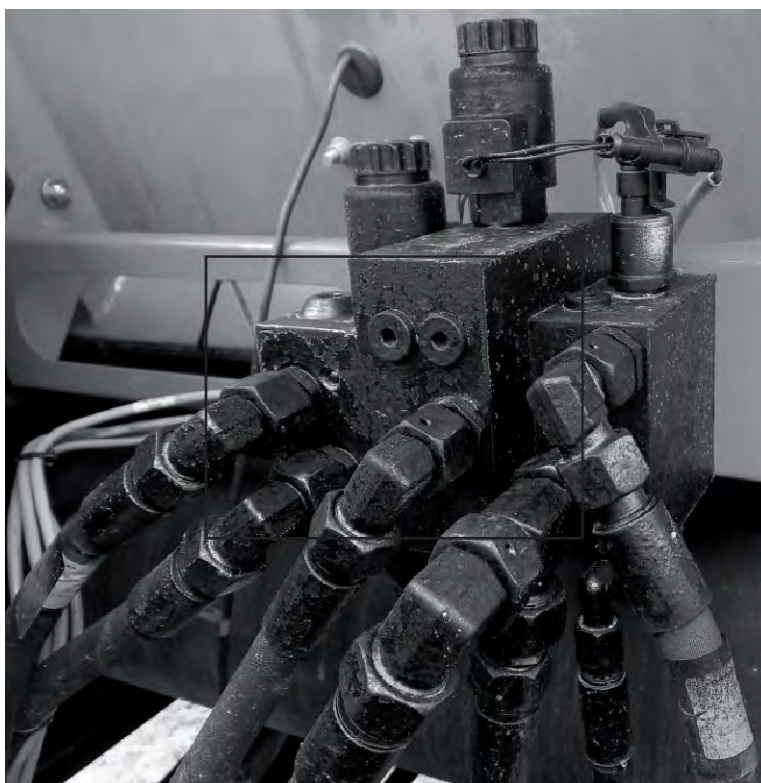
Obr. 69: Řídící blok
