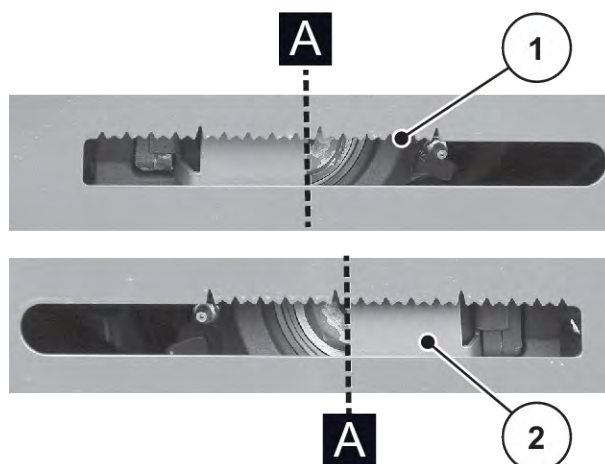
Obr. 79: Nastavení souprav talířových pružin
