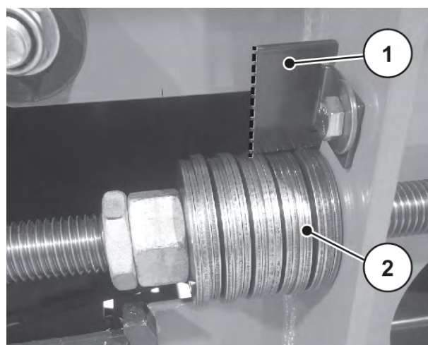
Obr. 78: Napnutí souprav talířových pružin
