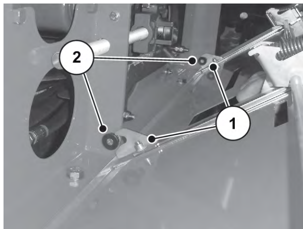
Obr. 57: Montáž bočního krytu
