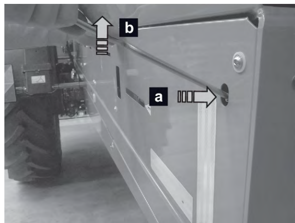
Obr. 55: Použití nastavovací páky
