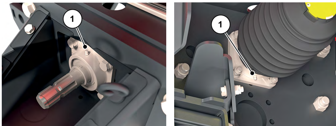
Obr. 63: Mazací místo průběžného pohonu kloubového hřídele
