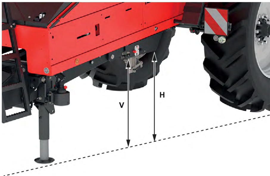
Obr. 74: Kontrola sklonu stroje
