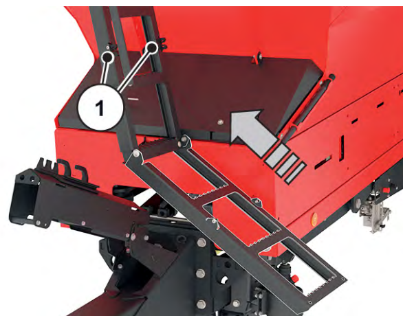
Obr. 36: Skládání žebříku
