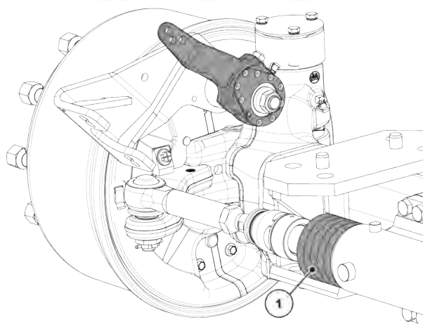
Obr. 72: Vymežovací podložky říditelné nápravy
