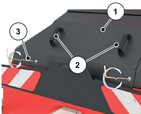
Obr. 68: Kryt rozmetacího mechanismu
