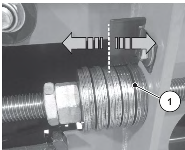
Obr. 80: Úprava souprav talířových pružin
