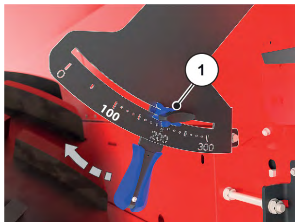
Obr. 37: Oblouk stupnice otevření předřazeného dávkovacího hradítka
