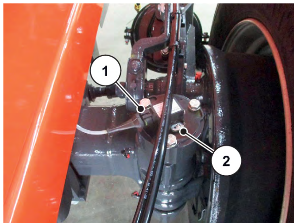
Obr. 73: Snímač úhlu nápravy
