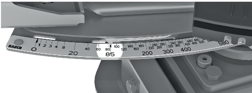
Obr. 45: Stupnice pro zobrazení rozmetaného množství
