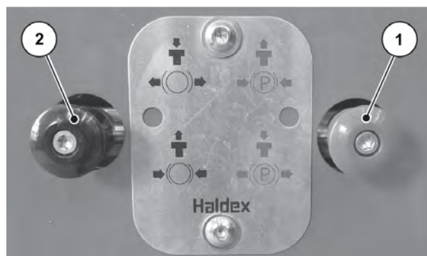
Obr. 48: Parkovací brzda (pneumatická brzdová soustava)
