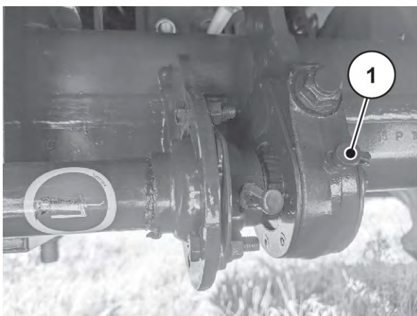
Obr. 65: Automatické seřizování páky brzdových klíčů tuhé nápravy
