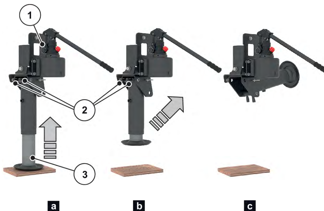
Obr. 27: Odklopení opěrné patky
