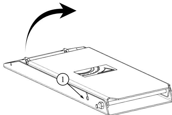
Obr. 50: Odklopení podkládacího klínu
