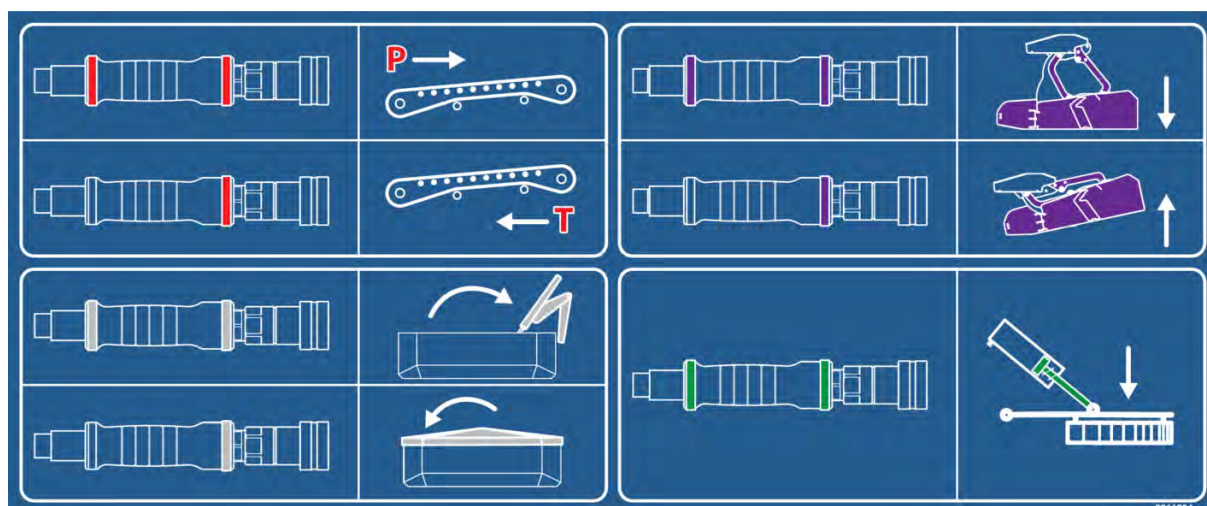
Fig. 24: Mærkning af hydraulikslangerne til basismaskinen/specialudstyr
