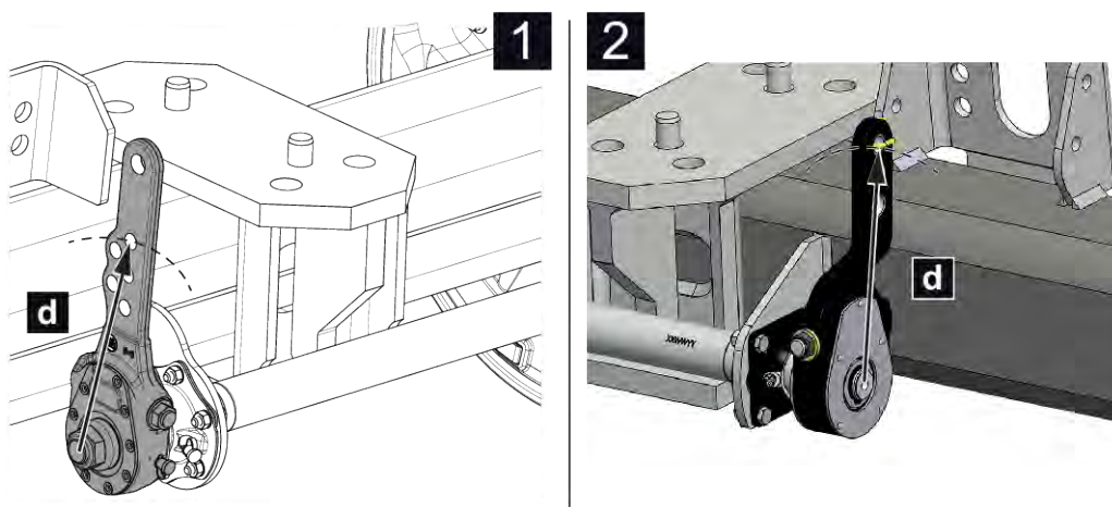
Fig. 69: Kontrollér tomkørselsvejen
