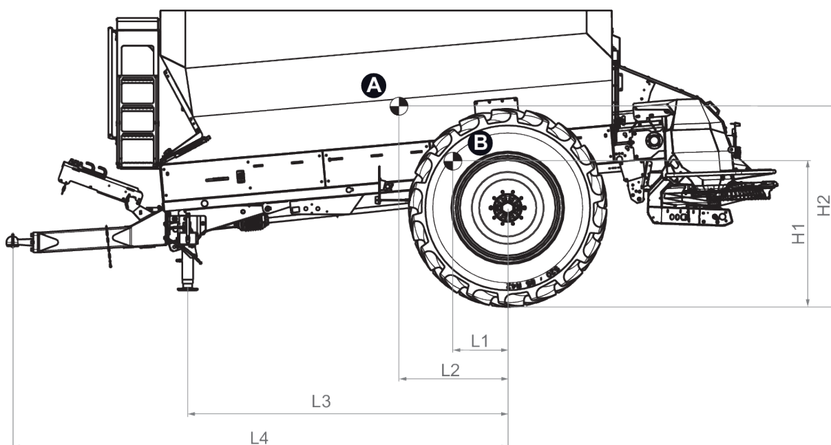
Fig. 14: Tyngdepunktets placering ved tilkobling fornedet
