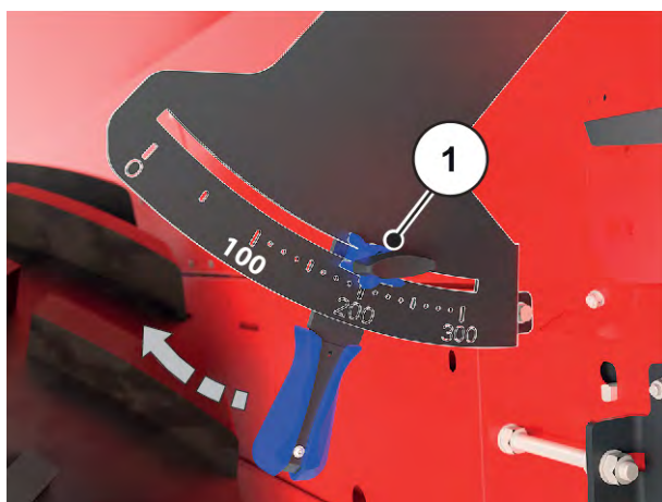
Fig. 33: Skalabue til fordoseringsspjæld-åbning
