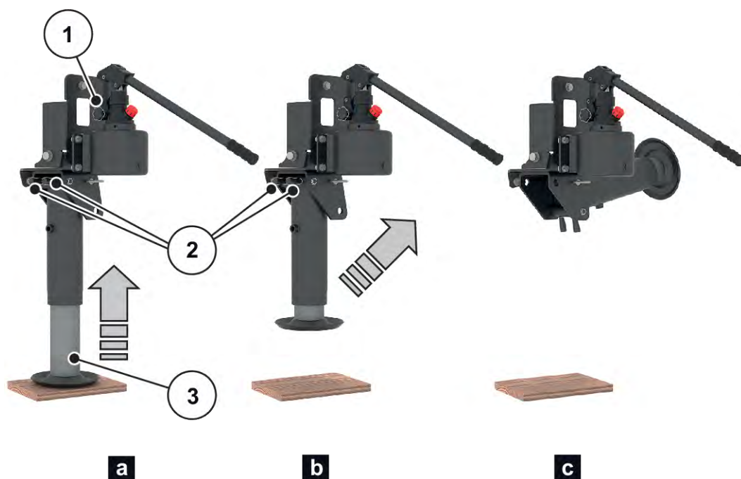
Fig. 25: Vækklapning af støttefod
