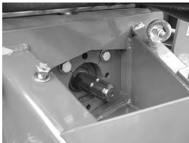
Fig. 18: Fedtsmøring af akseltappen
