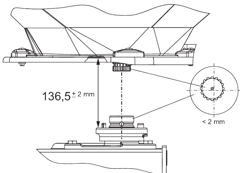
Fig. 80: Kontrol af position for spredeskivenav
