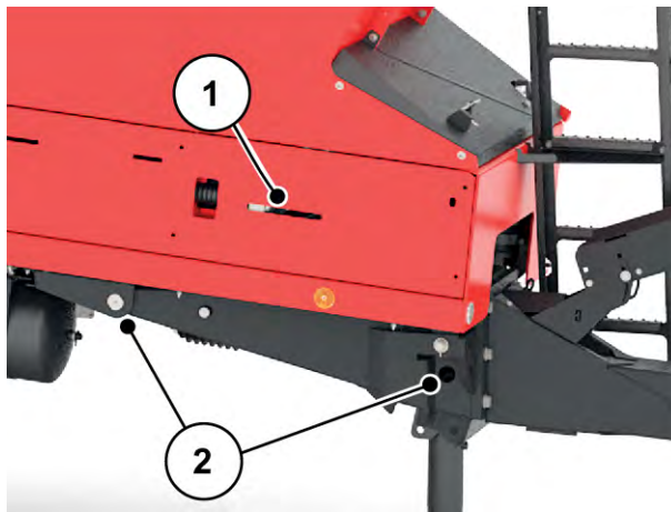
Fig. 77: Smørested for bånddrev og vognstang
