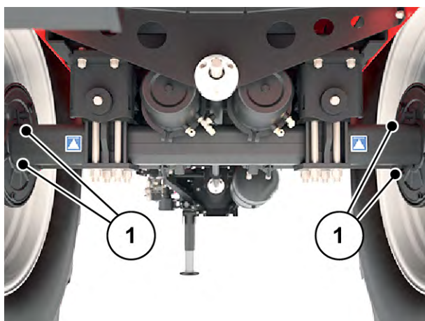
Fig. 76: Bremseforbindelsesled og aksel
