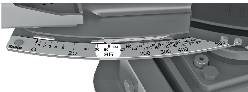
Fig. 41: Skala til visning af udbringningsmængden
