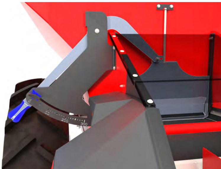
Fig. 29: Fordoseringsspjæld i lukket stilling
