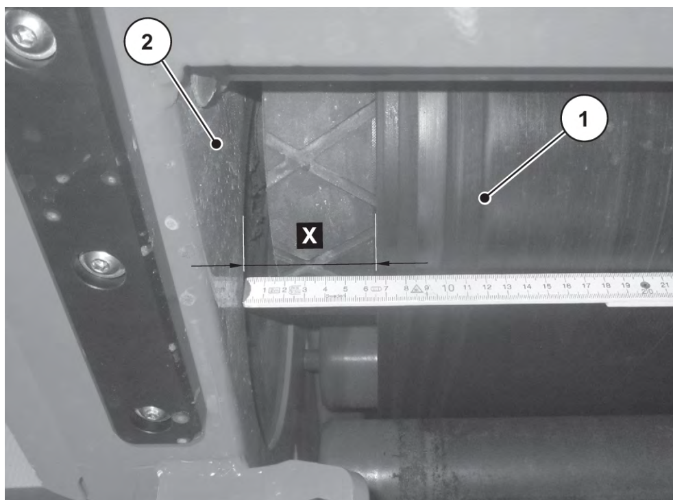
Fig. 59: Kontrol af transportbåndets position
