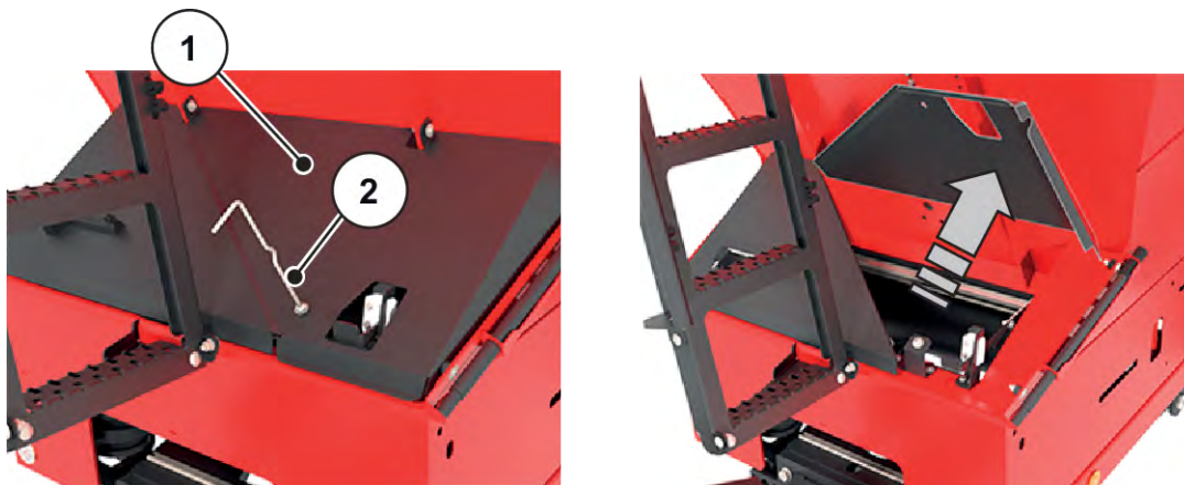
Fig. 53: Åbning af forreste afdækning
