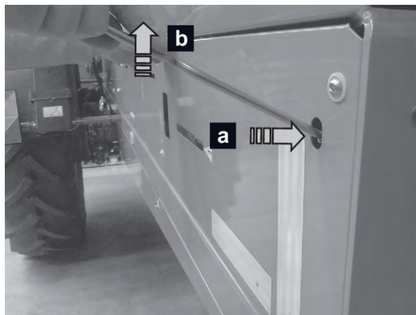
Fig. 49: Anvendelse af indstillingshåndtaget
