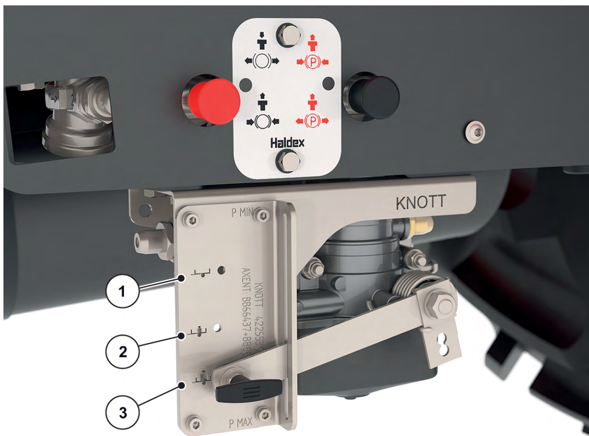
Fig. 27: Indstilling af bremsekraftfordeleren
