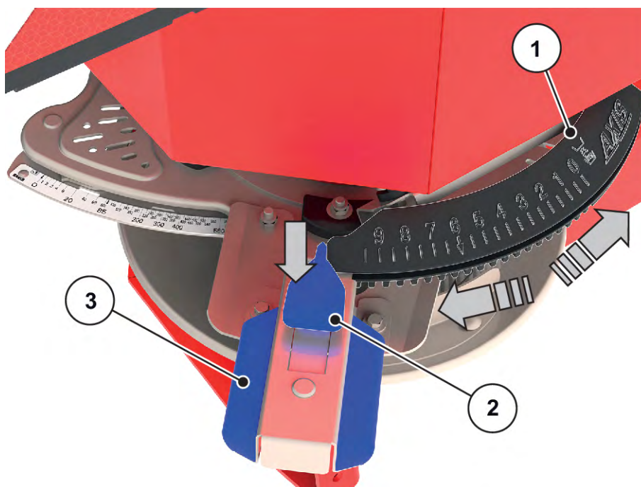
Fig. 40: Indstillingscenter for udbringningspunkt
