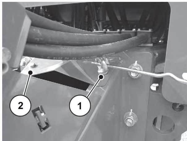
Fig. 17: Afmontering af beskyttelsesskærmen
