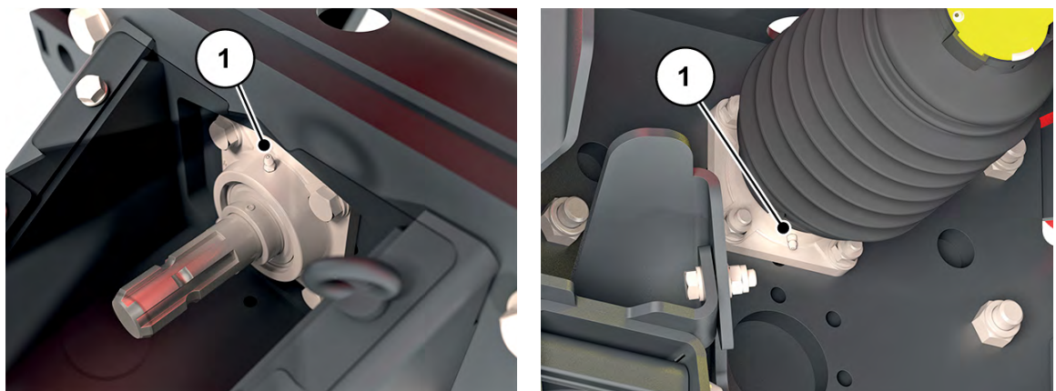
Fig. 79: Smørested på gennemgående kardanaksel
