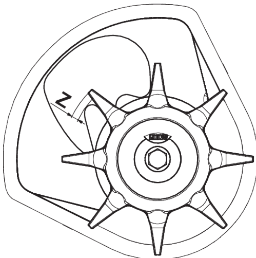
Fig. 82: Rørehovedets slitageområde
