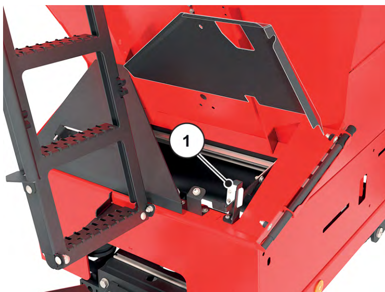
Fig. 30: Renselem i lukket stilling, foran i kørselsretning
