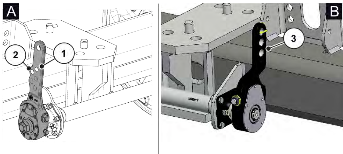
Fig. 72: Placering af forbindelsen bremsehåndtag/bremsecylinder
