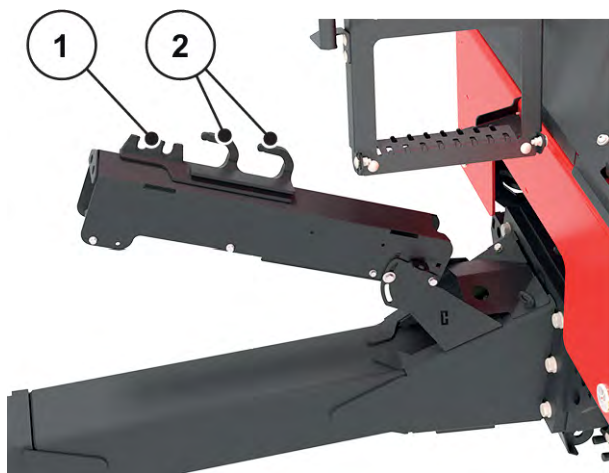
Fig. 48: Konsol til opbevaring af kabler, hydraulikslanger og pneumatikledninger
