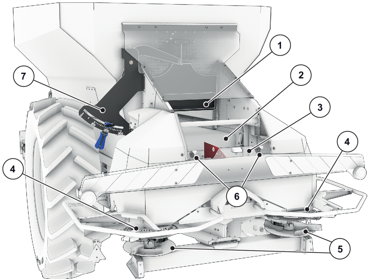
Ilust. 10: Vista general de módulos: Parte trasera
