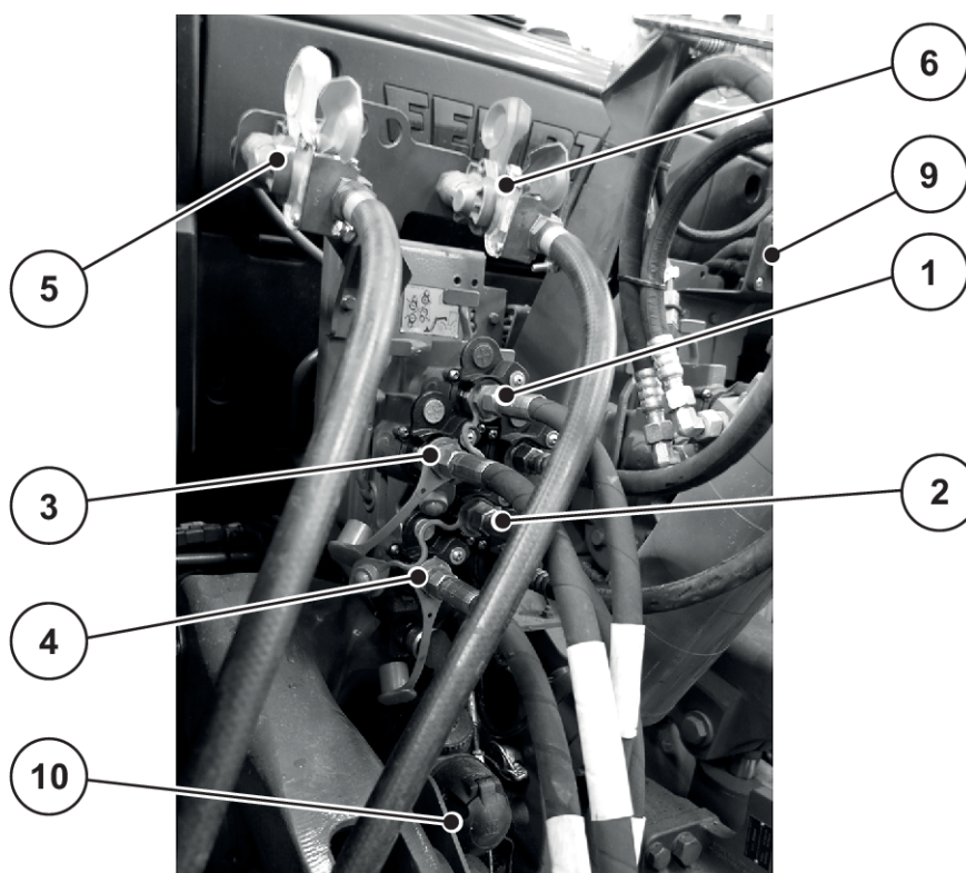
Ilust. 22: Orden de conexión de los conductos de la máquina en el tractor
