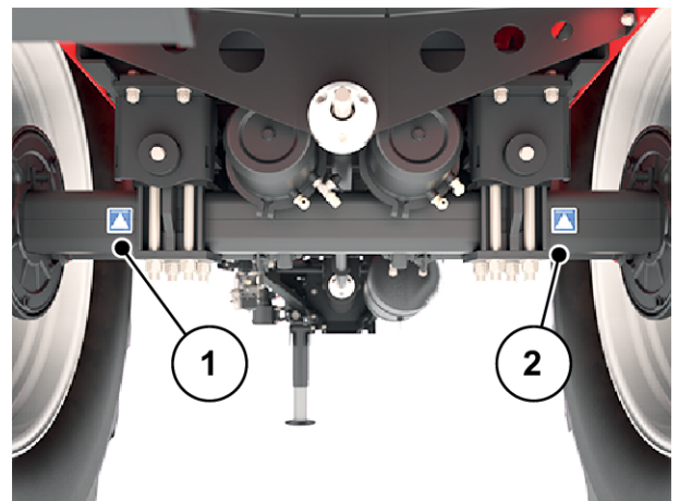
Ilust. 71: Puntos de colocación del gato
