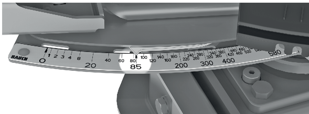
Ilust. 41: Escala para la visualización de la cantidad de dispersión
