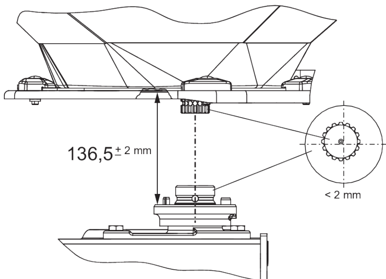
Ilust. 80: Comprobación de la posición del cubo de disco de dispersión
