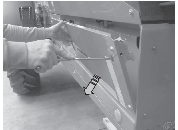
Ilust. 50: Apertura de la cubierta lateral
