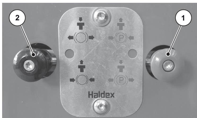
Ilust. 26: Freno neumático
