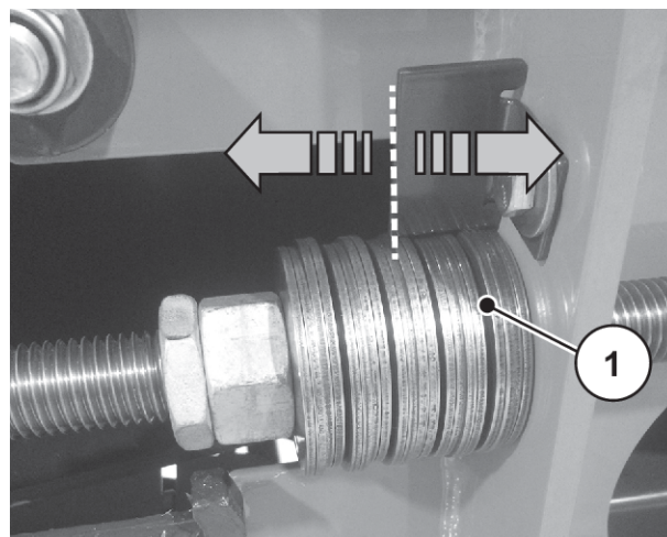
Ilust. 63: Desplazamiento de los bloques de muelles de disco
