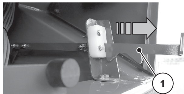
Ilust. 52: Palanca de la trampilla de limpieza
