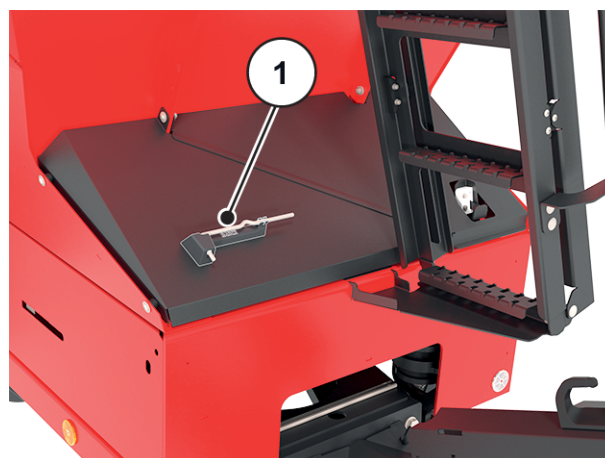
Ilust. 37: Ubicación de la palanca de ajuste
