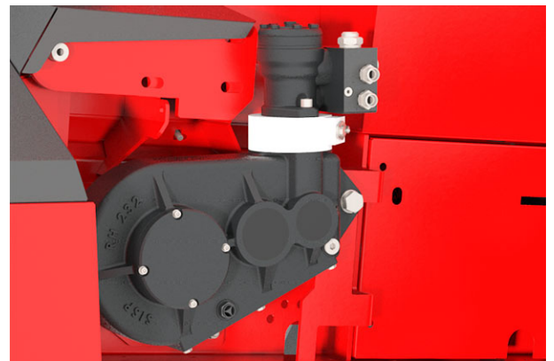
Ilust. 56: Comprobación del motor y del bloque hidráulico del accionamiento de la cinta transportadora
