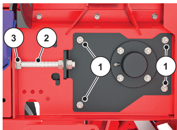
Ilust. 60: Posición del rodillo de accionamiento
