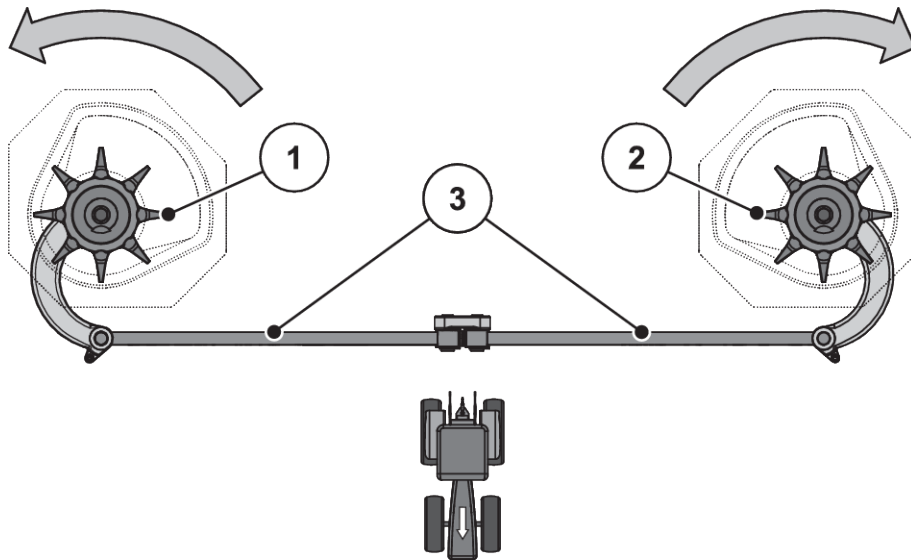
Ilust. 81: Comprobación del accionamiento del mecanismo agitador
