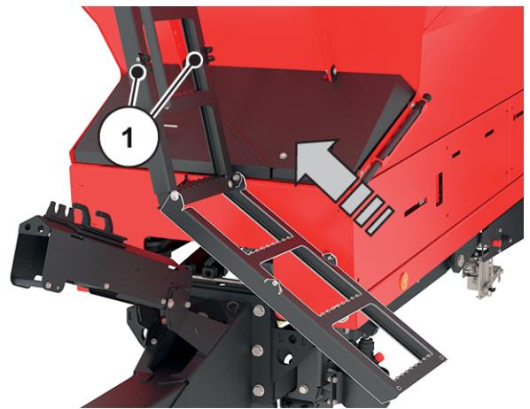
Ilust. 32: Plegar la escalera
