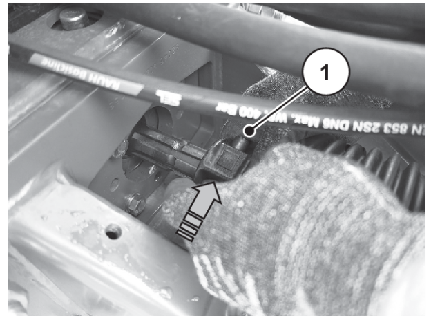
Ilust. 19: Inserte el eje articulado en el muñón de engranaje
