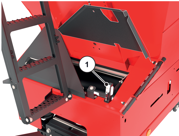
Ilust. 30: Trampilla de limpieza en posición cerrada, en la parte delantera en el sentido de la marcha
