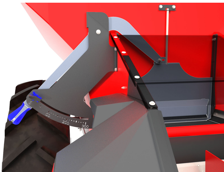
Ilust. 29: Corredera de dosificación previa en posición cerrada
