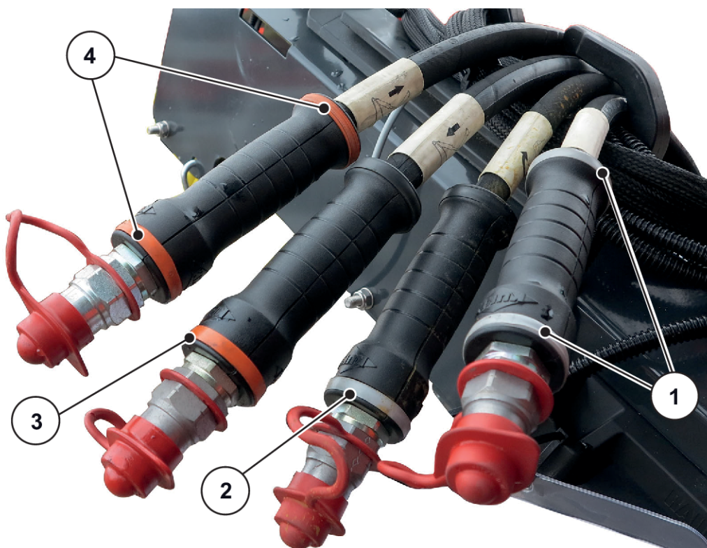
Ilust. 23: Identificación de las mangueras hidráulicas
