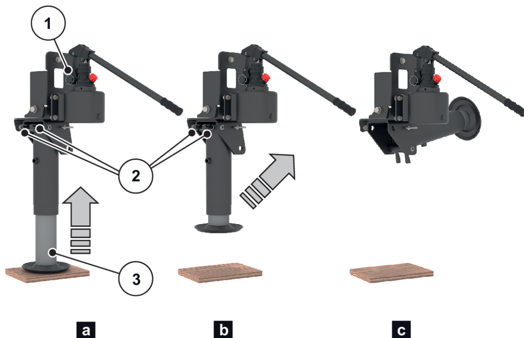
Ilust. 25: Retraer el pie de apoyo
