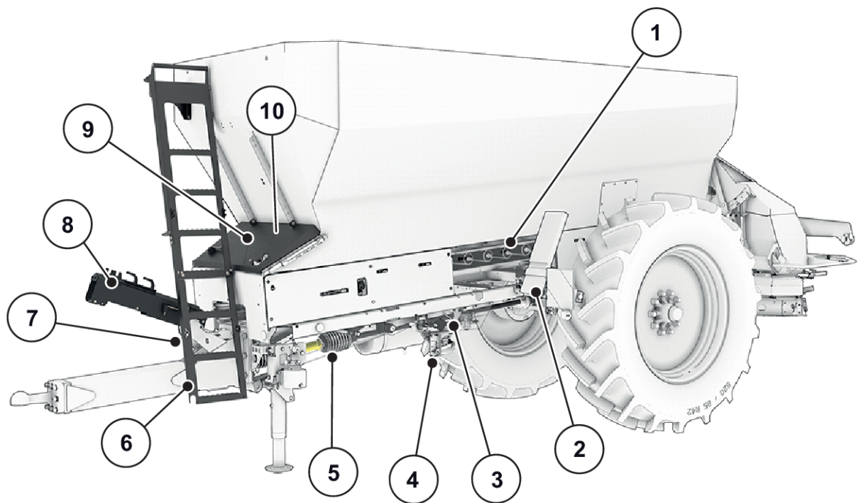
Ilust. 9: Vista general de módulos: Parte delantera
