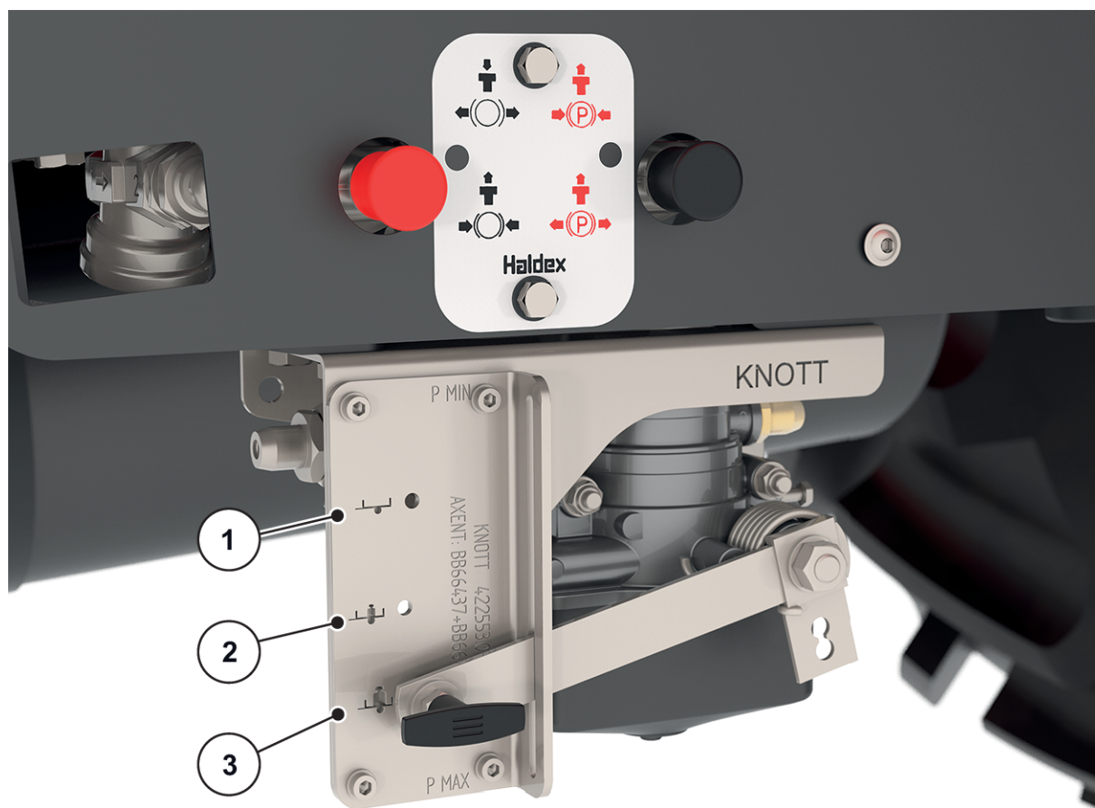
Ilust. 27: Ajuste del regulador de la fuerza de frenado
