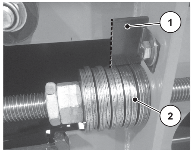
Ilust. 61: Volver a tensar los bloques de muelles de disco
