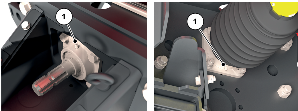
Ilust. 79: Punto de lubricación del accionamiento de los ejes articulados
