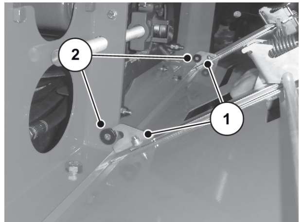
Ilust. 51: Montaje de la cubierta lateral
