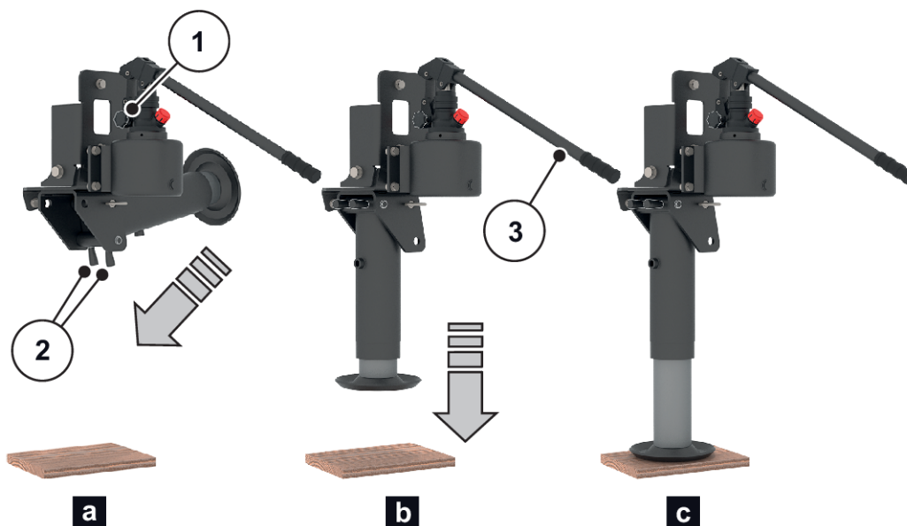
Ilust. 47: Extraer el pie de apoyo
