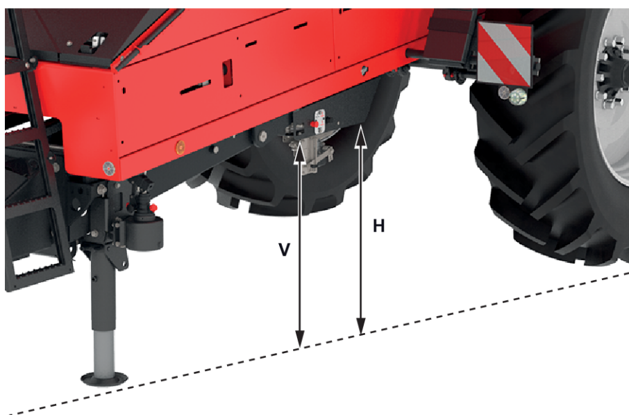
Ilust. 57: Comprobación de la inclinación de la máquina
