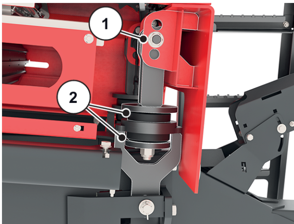
Ilust. 58: Comprobación de la suspensión de la barra
