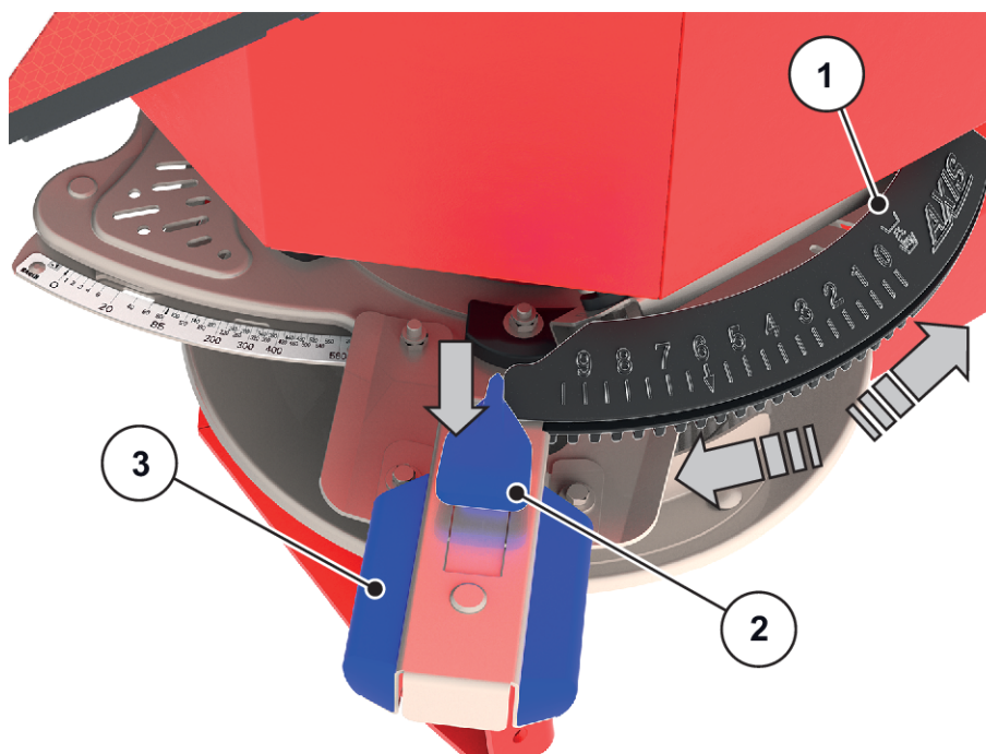
Ilust. 40: Centro de ajuste del punto de salida
