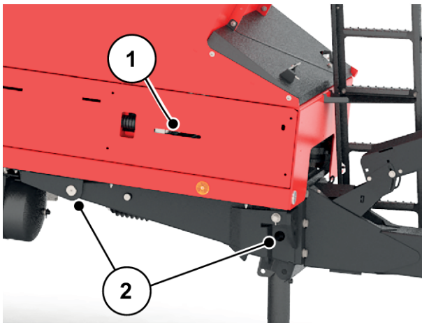
Ilust. 77: Punto de lubricación del accionamiento de cinta y de la barra
