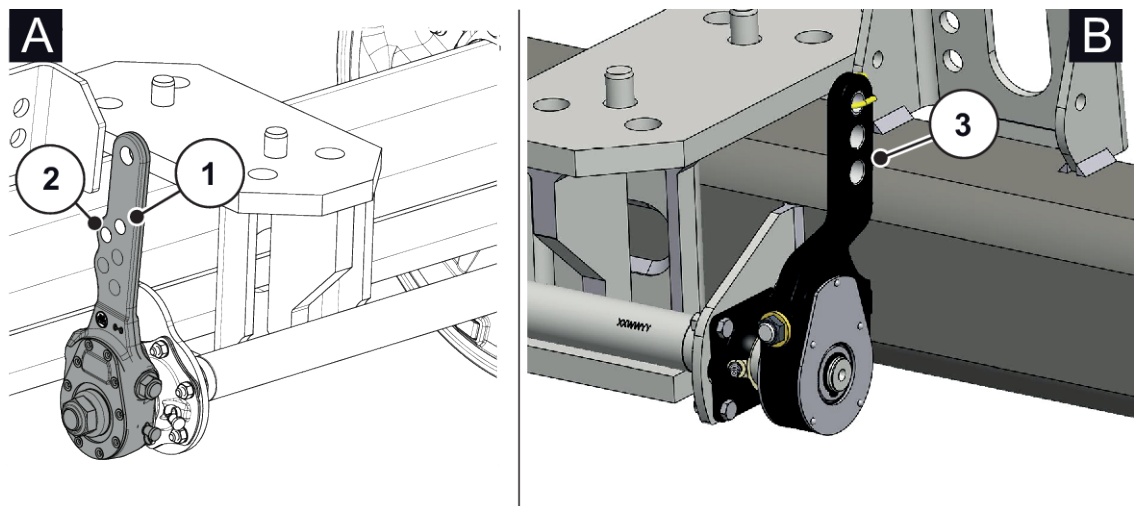
Ilust. 72: Posición de la unión de palanca de freno/cilindro de freno
