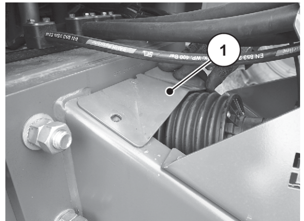
Ilust. 20: Montaje de la chapa protectora
