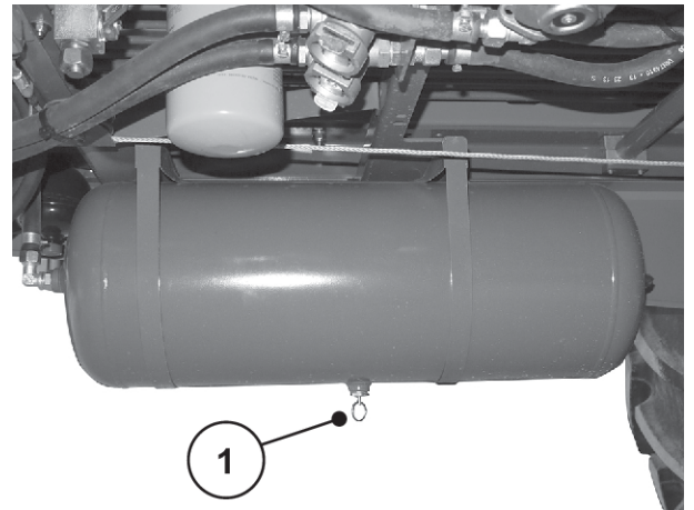
Ilust. 70: Drenaje del depósito de aire
