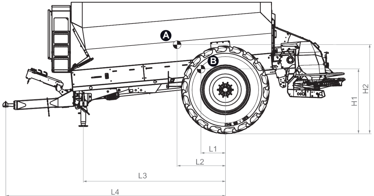
Ilust. 14: Ubicación del centro de gravedad en el enganche inferior
