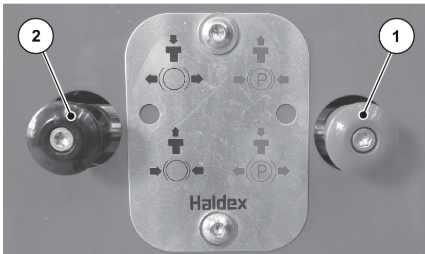
Ilust. 28: Liberación del freno de estacionamiento
