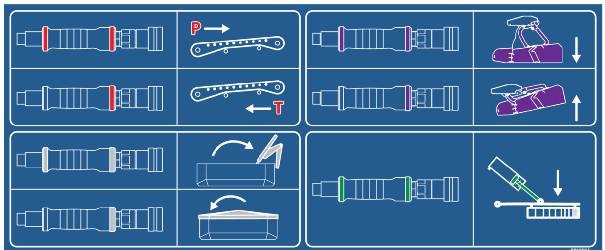
Ilust. 24: Identificación de las mangueras hidráulicas en la máquina básica/equipamientos especiales
