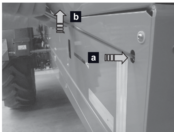
Ilust. 49: Uso de la palanca de ajuste
