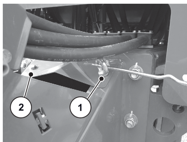
Ilust. 17: Extracción de la chapa protectora
