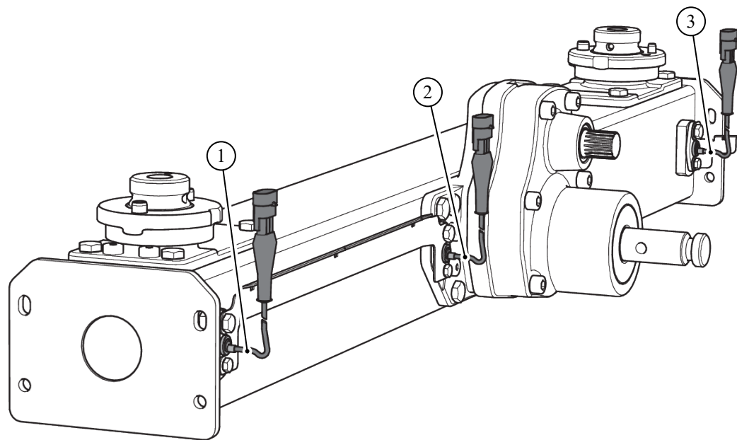
Ilust. 13: Regulación del flujo másico mediante medición del par de giro de los discos de dispersión
