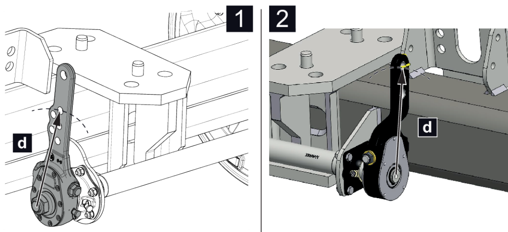
Ilust. 69: Comprobación del trayecto en vacío
