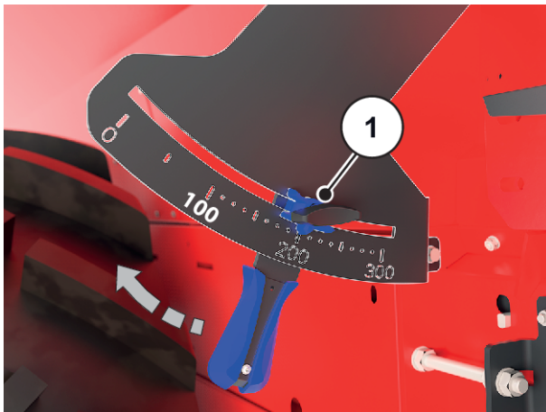
Ilust. 33: Rueda graduada para la apertura de la corredera de dosificación previa
