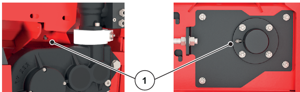
Ilust. 78: Punto de lubricación del accionamiento de cinta transportadora
