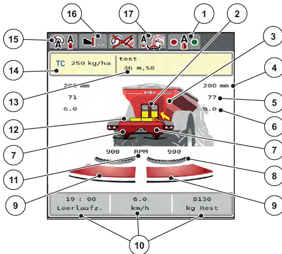
Fig. 1: Maskinstyringens display
