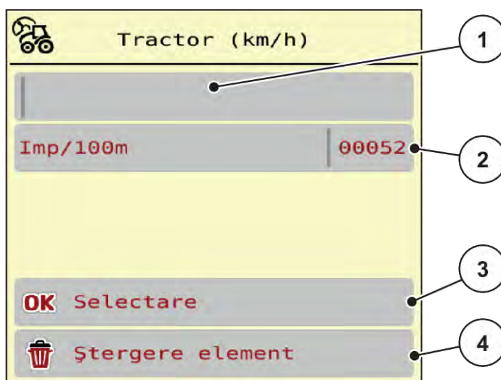
Fig. 26: Profil tractor
