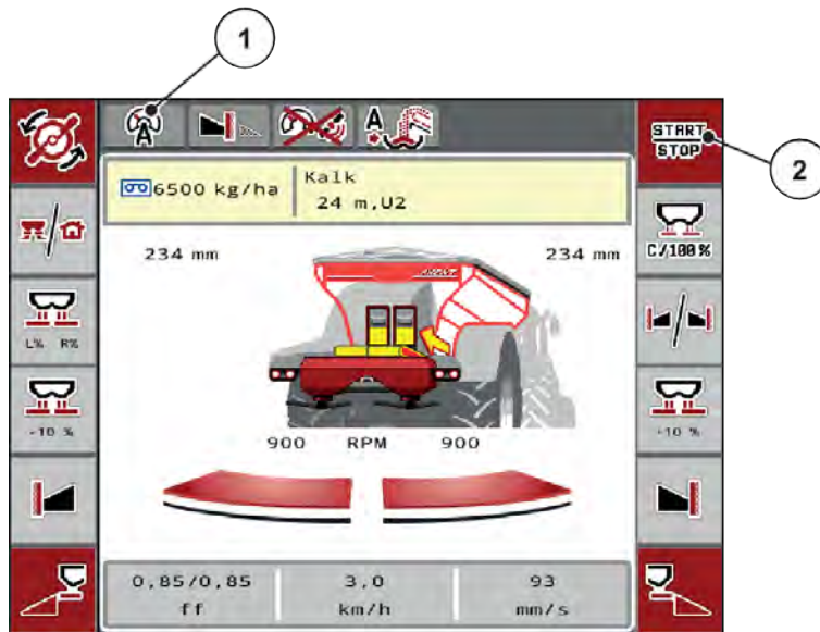
Рис. 53: Рабочий экран при работе с известью
