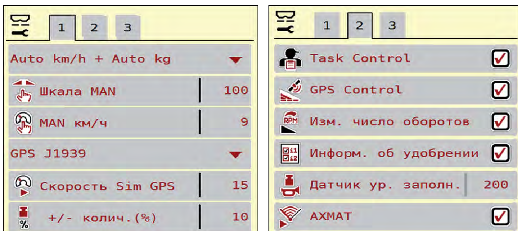
Рис. 21: Меню Настройки машины, вкладки 1 и 2
