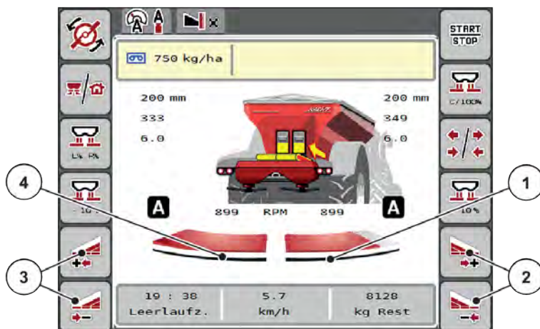
Рис. 44: Рабочий экран: Секции рабочей ширины с 2 секциями рабочей ширины
