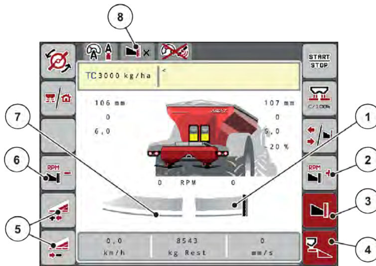
Рис. 46: Рабочий экран: одна секция рабочей ширины слева и режим для внесения на границе поля справа
