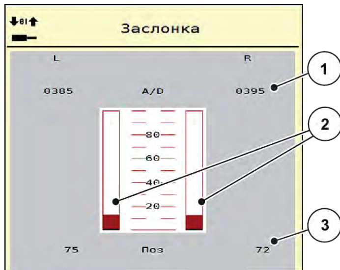
Рис. 32: Тест/диагностика; пример: Заслонка
