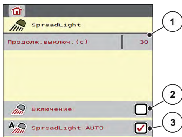
Рис. 37: Меню SpreadLight
