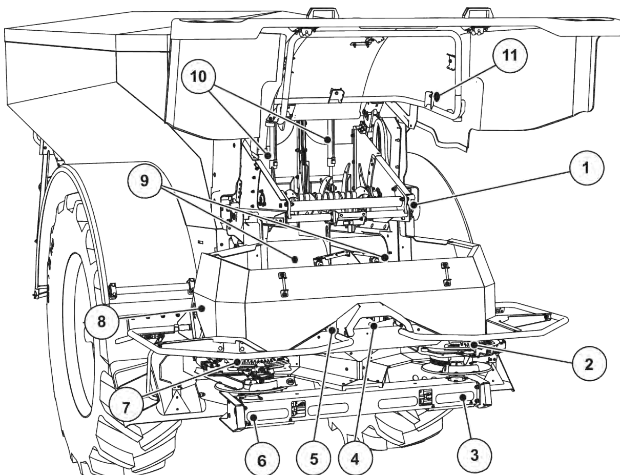
Rys. 6: Przegląd urządzeń wykonawczych i czujników w rozrzutniku wielkopowierzchniowym AXENT i rozrzutniku nawozu AXIS-PowerPack
