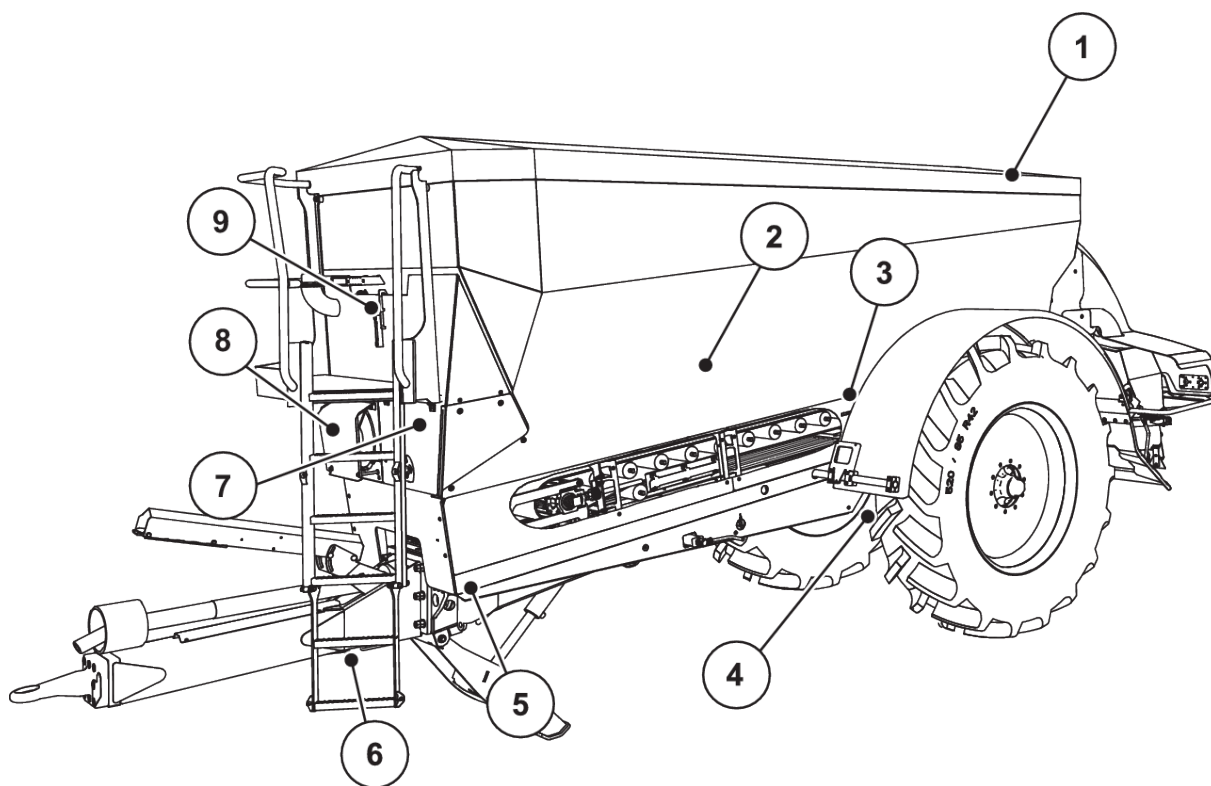
Ilust. 5: Vista general de los actuadores y sensores en la abonadora de gran superficie AXENT
