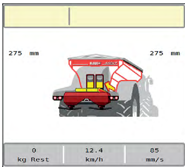
Fig. 8: Niveauidikator AXENT-beholder
