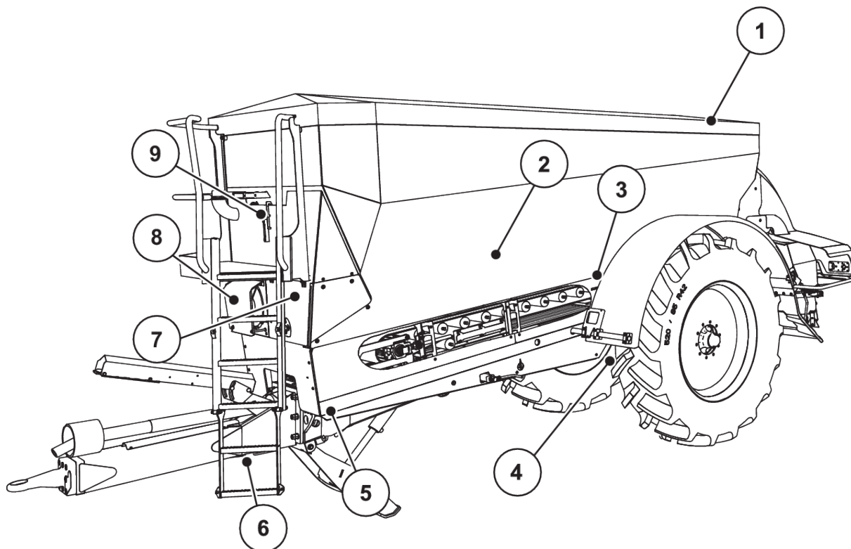
Fig. 5: Oversigt over aktuatorer og sensorer på spredemaskinen AXENT
