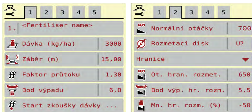
Obr. 18: Menu Nastavení hnojiva, režim rozmetání vápna, záložka 1 a 2
