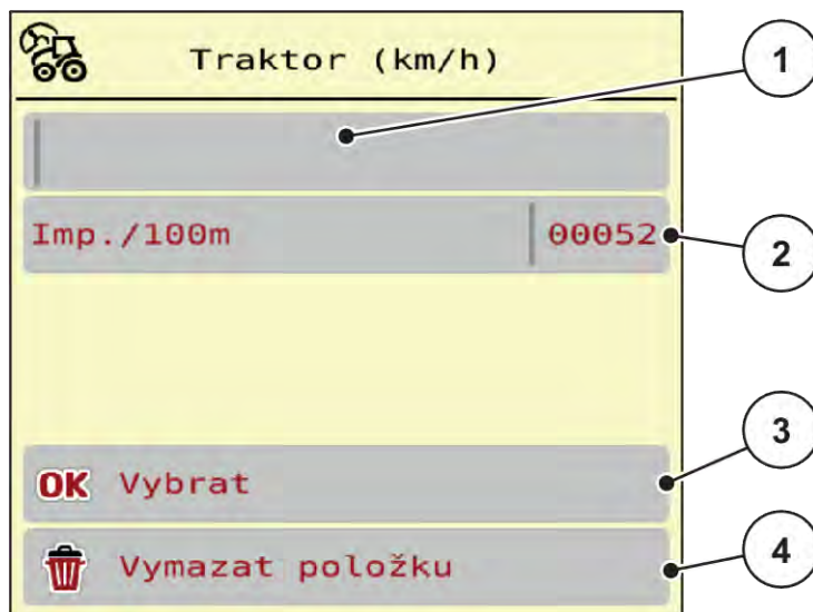
Obr. 25: Profil traktoru
