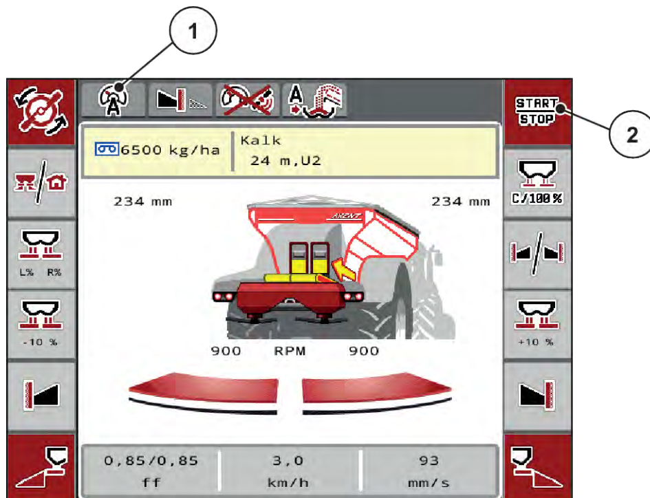
Obr. 52: Provozní obrazovka v provozním režimu rozmetání vápna
