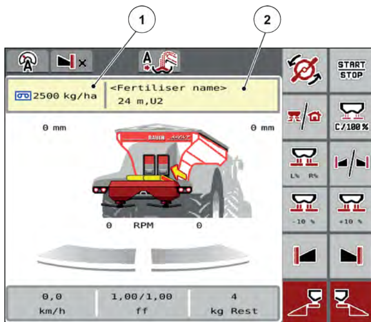
Obr. 19: Zadání dávky na dotykové obrazovce
