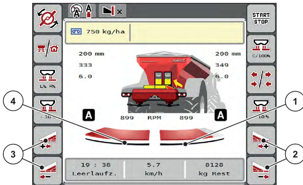
Obr. 43: Provozní obrazovka: Dílčí záběry se 2 dílčími záběry
