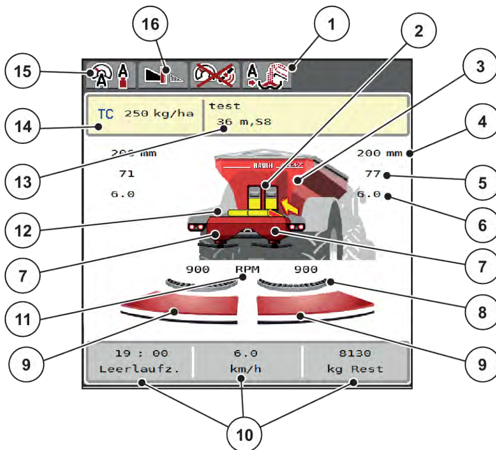
Obr. 1: Displej ovládání stroje
