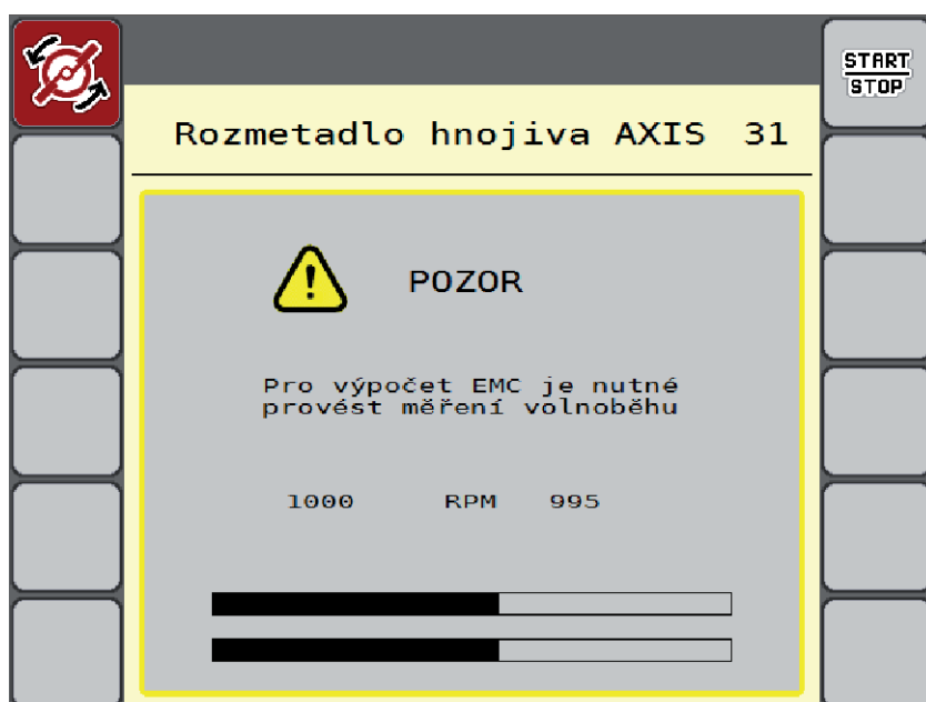
Obr. 46: Alarmová signalizace měření vyprázdnění
