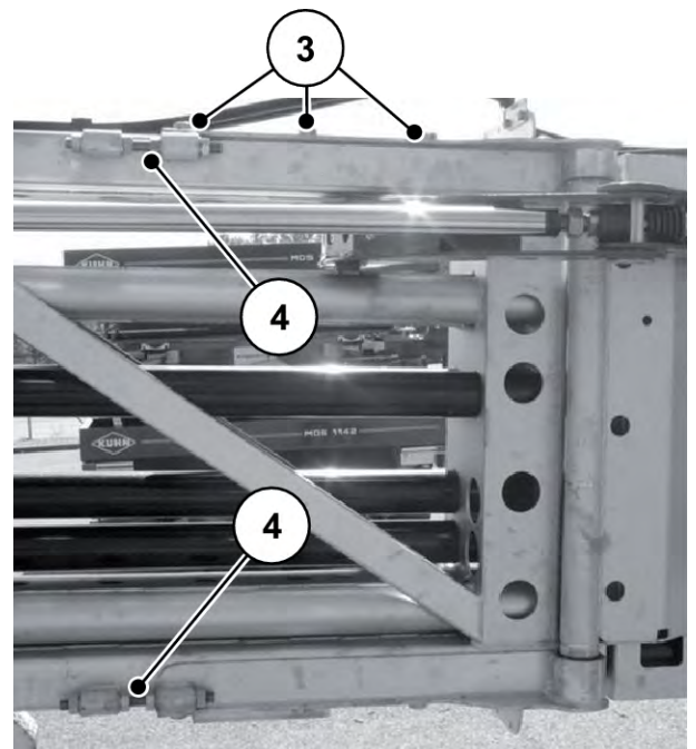
Afb. 60: Uitgeklapte armsegmenten horizontaal instellen
