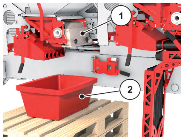
Afb. 40: Opvangbak voor meststof onder de doseerinrichting
