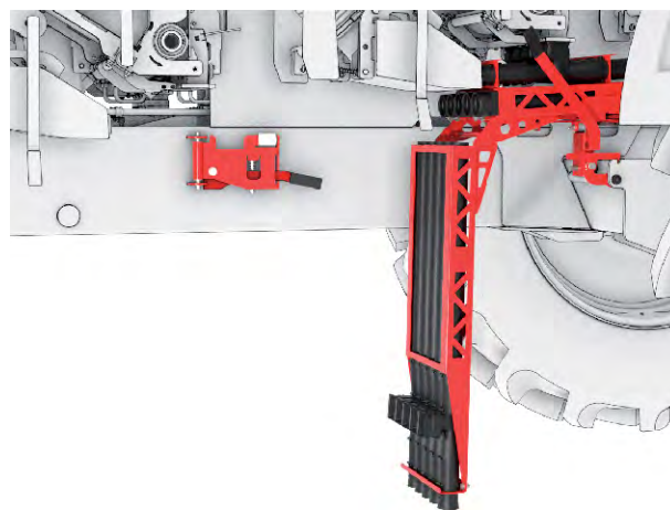
Afb. 39: Luchtgeleiding aftappen
