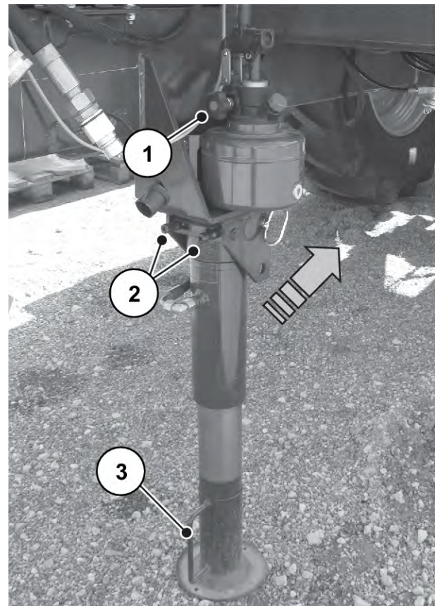
Afb. 25: Steunvoet wegklappen
