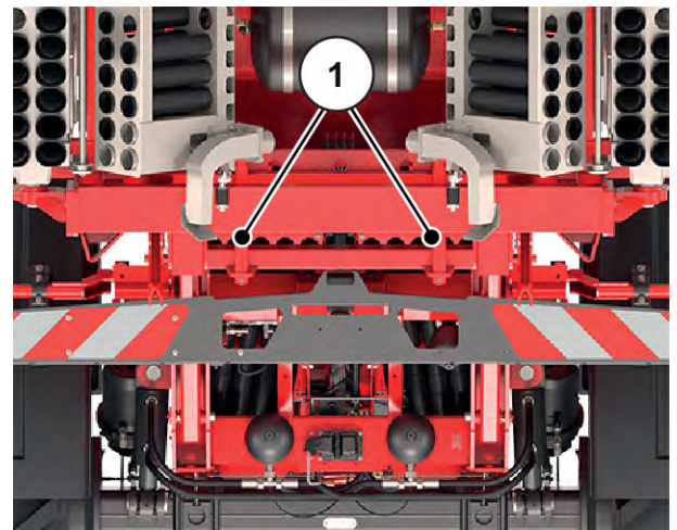
Afb. 92: Glijvlak tussen geleidingsbout en slingerframe
