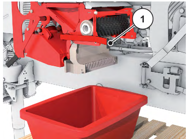
Afb. 52: Strooibak eronder plaatsen
