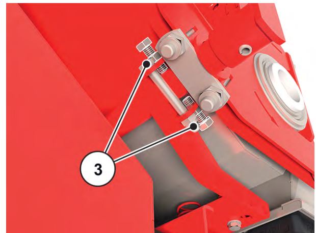
Afb. 58: Afstand nokkenwielen - strooibak instellen
