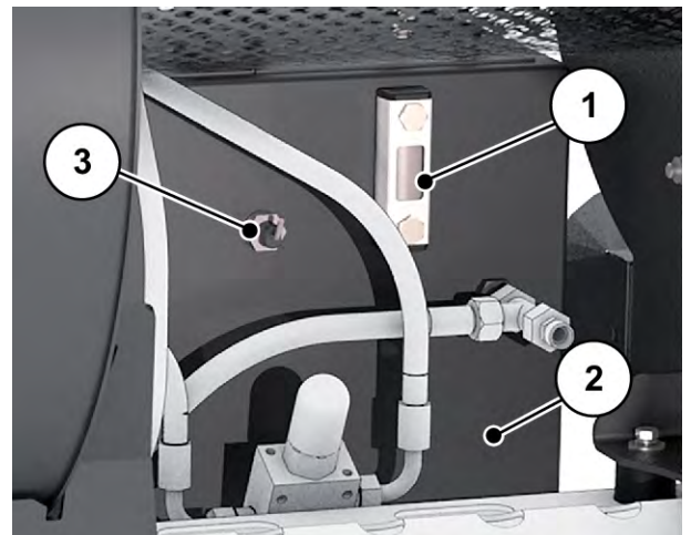
Afb. 76: Positie olietank vario-aandrijving
