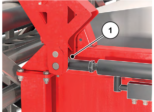
Afb. 94: Hydrocilinder voor borging van de arm
