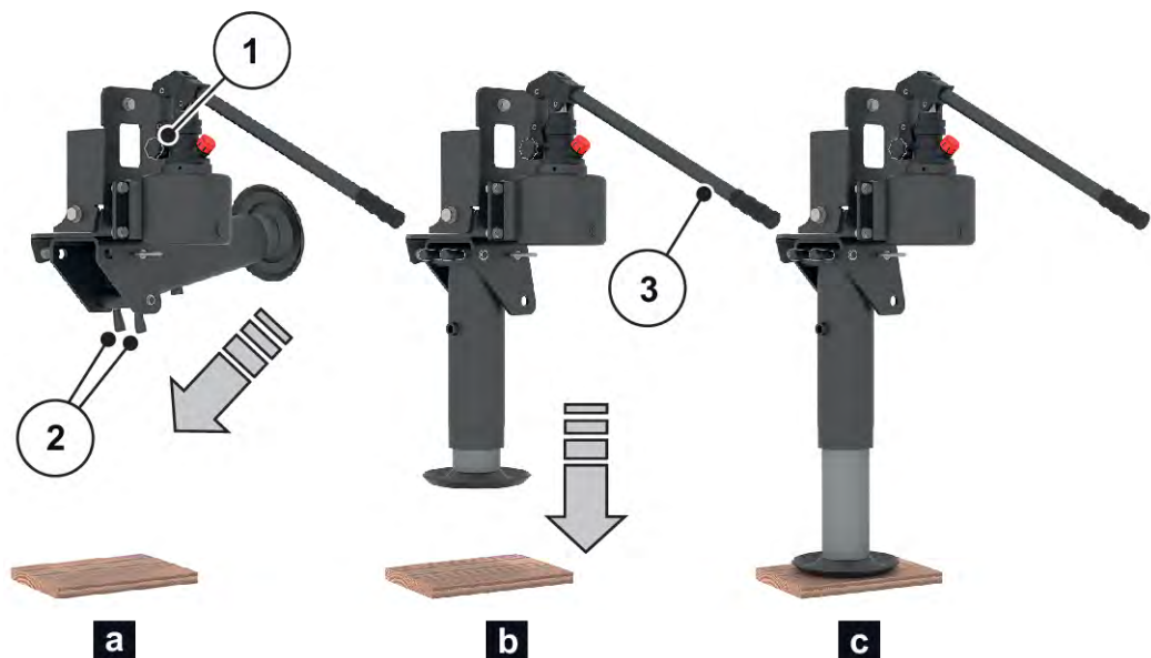
Afb. 56: Steunvoet uitschuiven
