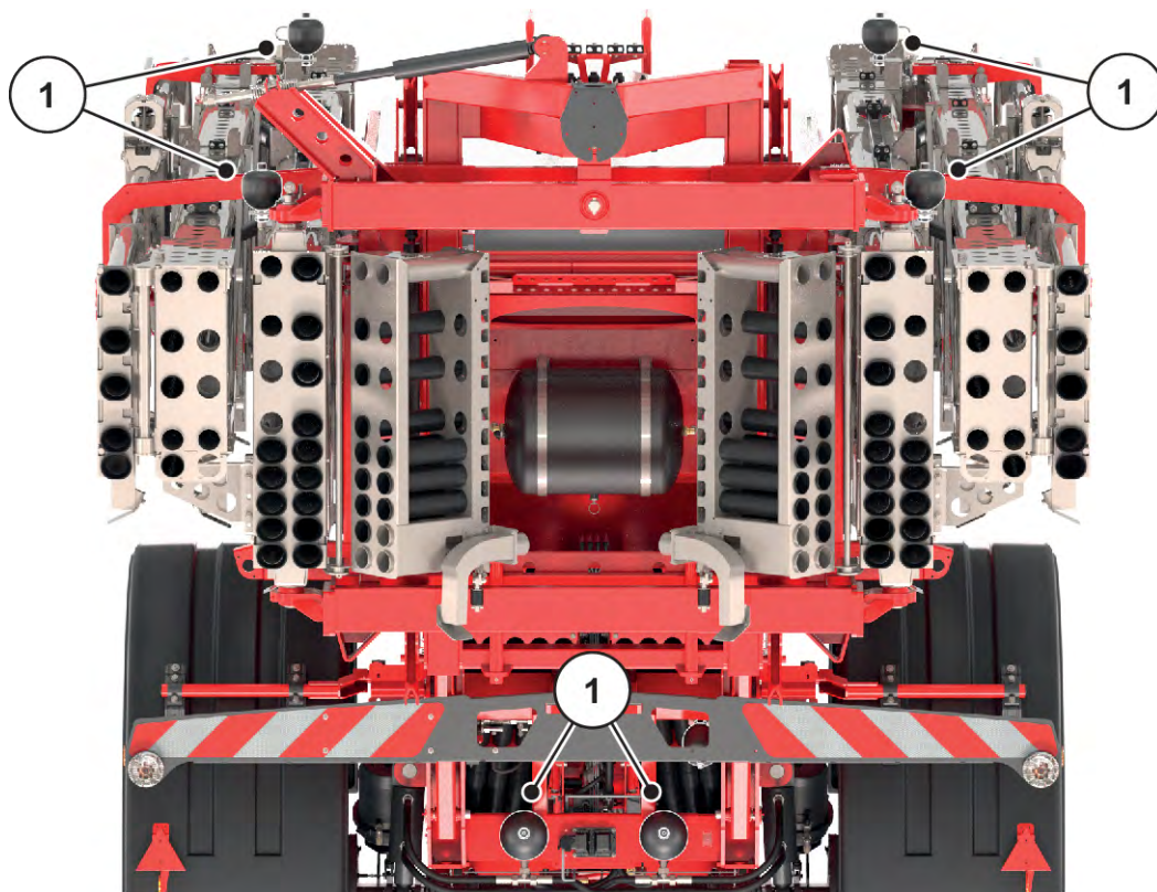
Afb. 72: Stikstofreservoirs
