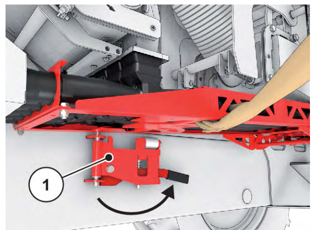
Afb. 38: Steun naar achteren zwenken
