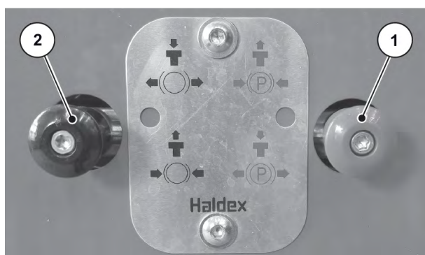
Afb. 43: Parkeerrem ontkoppelen
