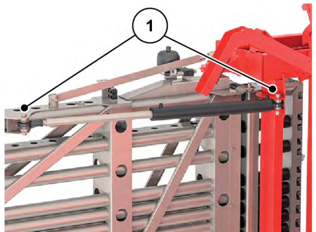
Afb. 95: Begindeel van de arm
