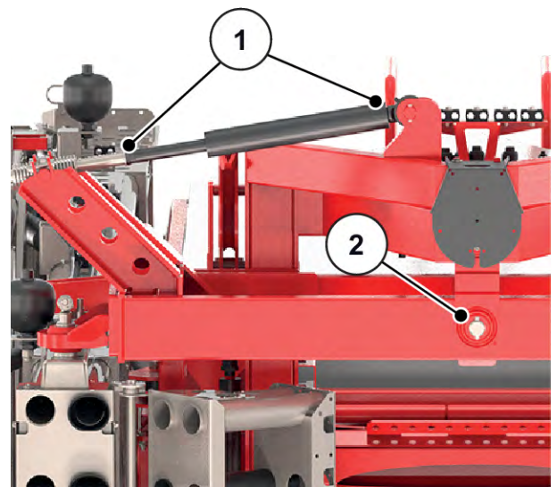
Afb. 91: Smeerpunten slingerframe
