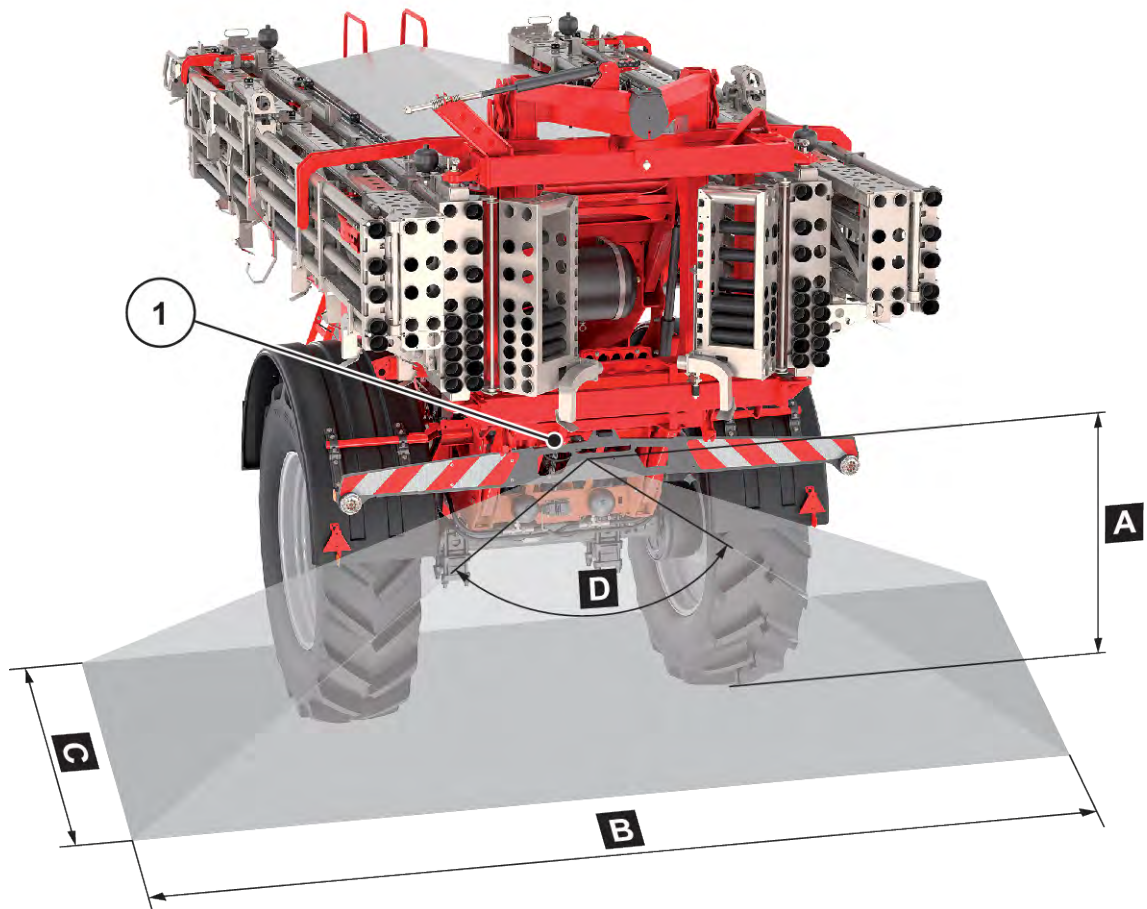
Afb. 33: Zichtveld achteruitrijcamera
