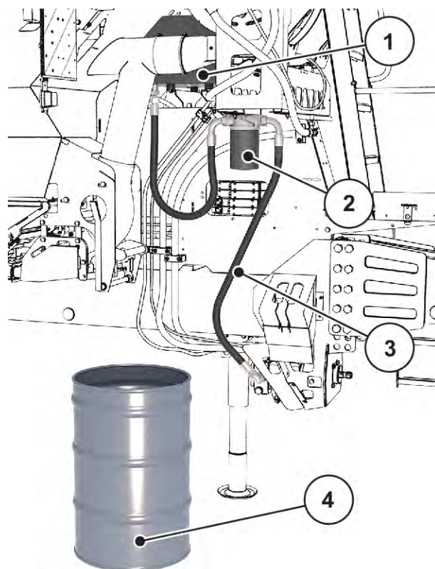
Afb. 78: Oliefilter
