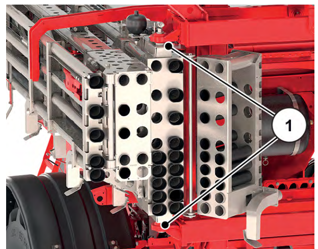
Afb. 93: Scharnierlager voor arm aan slingerframe
