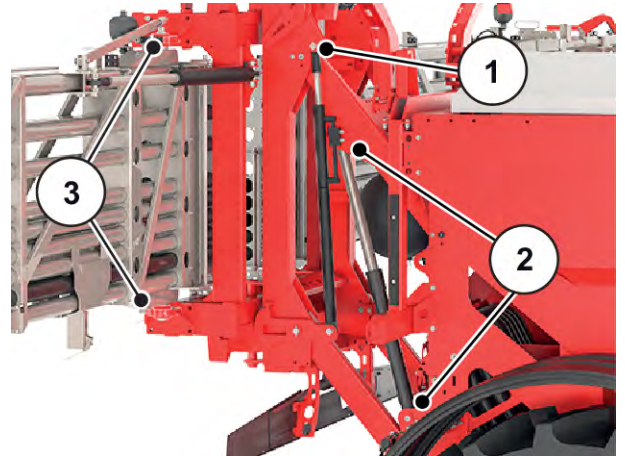
Afb. 99: Scharnierlager aan de hydrocilinder voor parallellogram
