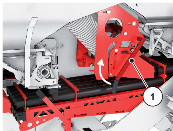
Afb. 49: Achterste drukkamer losmaken
